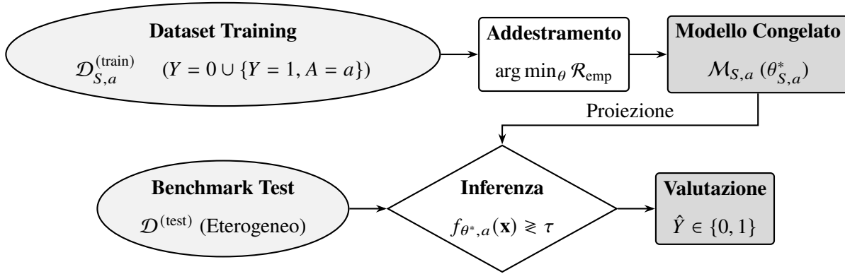
Figura 3.4: Flusso concettuale del protocollo di valutazione incrociata ( cross-evaluation ). Il modello specialistico \mathcal{M}_{S,a} , addestrato esclusivamente sulla singola minaccia a , viene congelato e proiettato in fase di inferenza sull'intero benchmark eterogeneo \mathcal{D}^{(\text{test})} .
