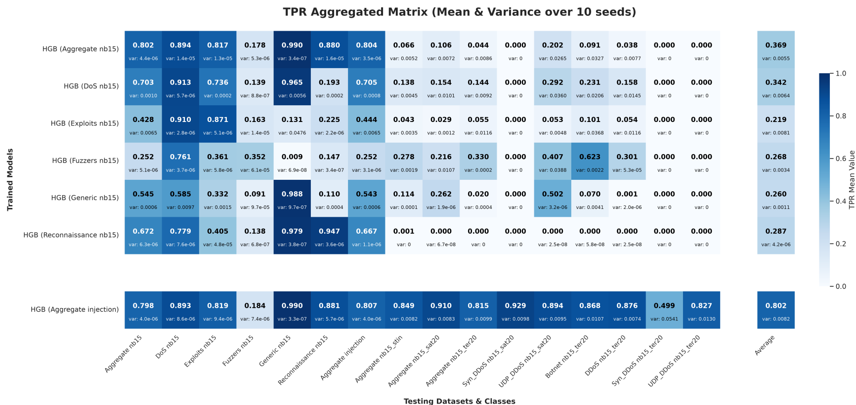
Figura A.2: Matrice aggregata della TPR per Histogram-based Gradient Boosting nel confronto tra modelli sorgente e baseline INJECTION.
