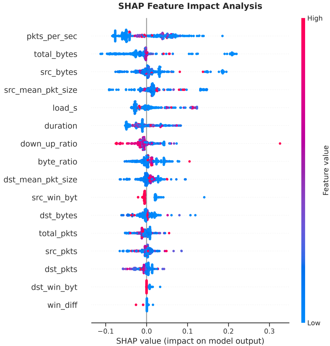
Figura 5.7: Summary plot SHAP della baseline INJ. implementata mediante Random Forest, valutata sul test set INJECTION con seed s = 42 .
