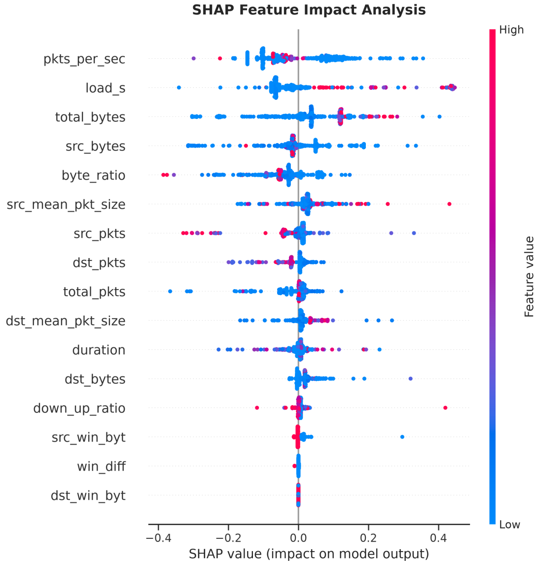
Figura 5.9: Summary plot SHAP della baseline INJ . implementata mediante Decision Tree, valutata sul test set INJECTION con seed s = 42 .
