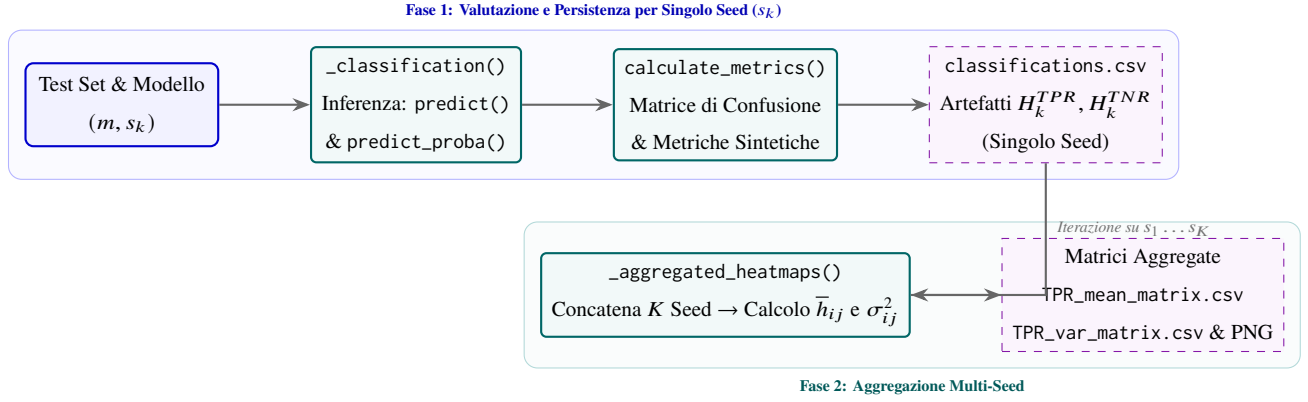
Figura 4.5: Pipeline a due stadi per il calcolo delle metriche di classificazione, tracciamento su file system e aggregazione statistica multi-seed.
