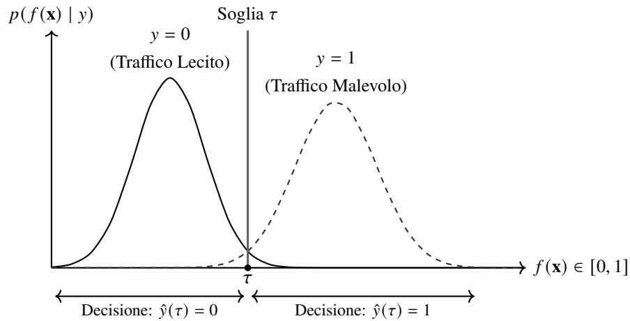
Figura 3.9: Mappatura della probabilità a posteriori f(\mathbf{x}) sulla regola decisionale binaria \hat{y}(\tau) in funzione della soglia \tau .
