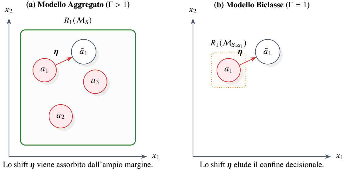
Figura 3.7: Rappresentazione bidimensionale nello spazio delle caratteristiche \mathcal{X} dell’impatto del domain shift (vettore di traslazione \eta ) a seconda della granularità del modello. A sinistra, la maggiore ampiezza spaziale del modello aggregato garantisce tolleranza generalista; a destra, l’ottimizzazione specialistica sul singolo supporto malevolo determina rigidità sotto perturbazione.
