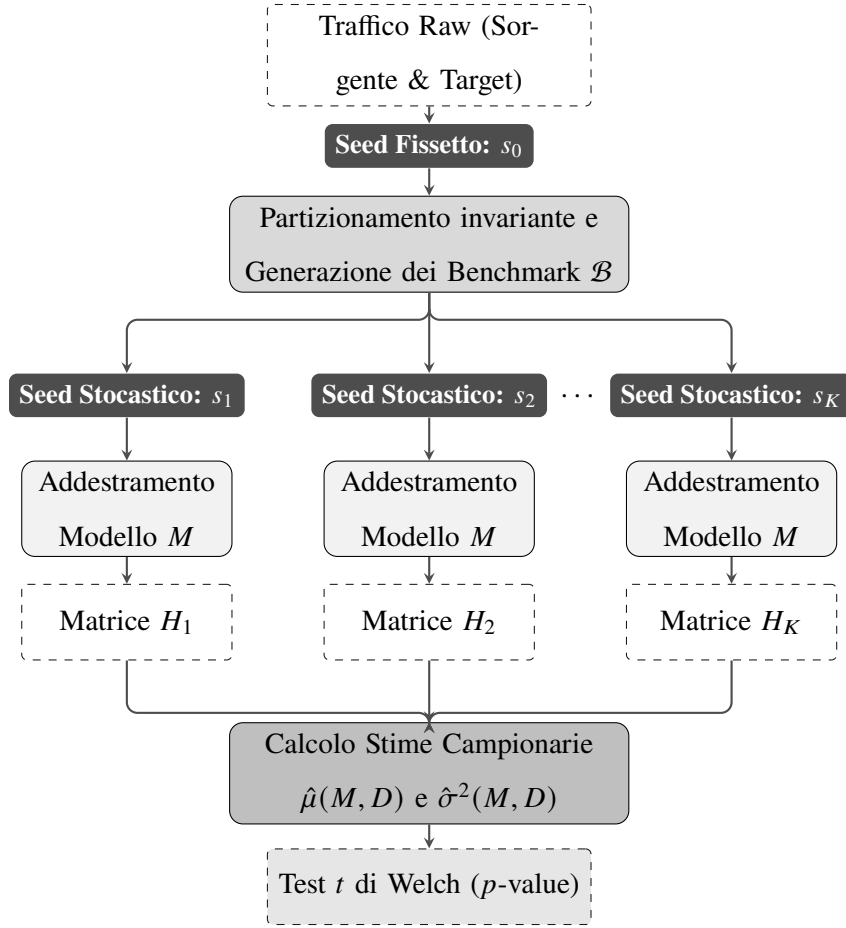
Figura 3.6: Diagramma di flusso del protocollo di isolamento e valutazione stocastica. La stabilità della partizione dei dati è forzata top-down dall'unico seed deterministico s_0 , delegando la totalità della varianza osservata tra le matrici H_k all'inizializzazione stocastica dettata dall'insieme dei seed S interni agli stimatori.
