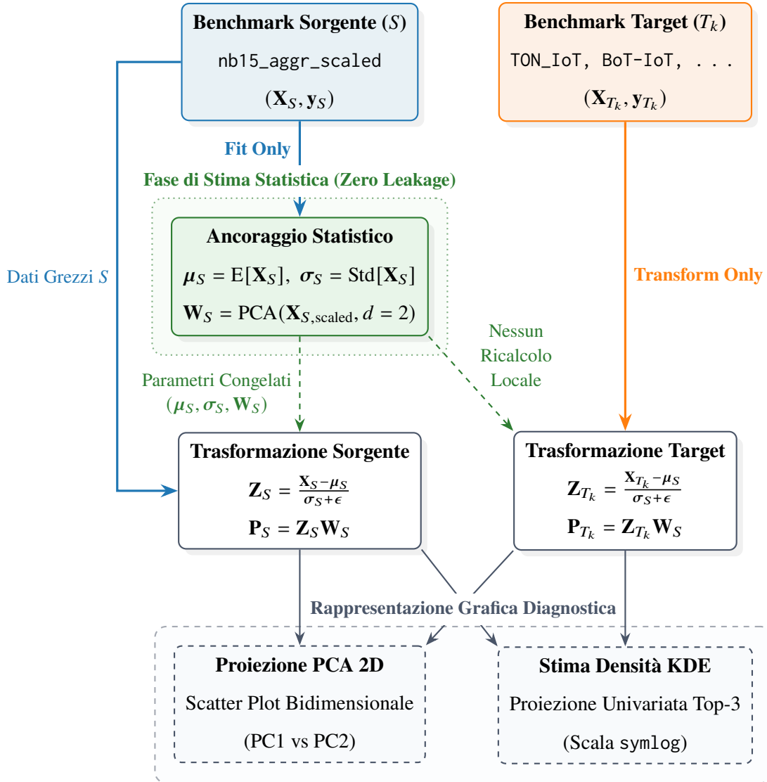
Figura 4.8: Schema concettuale della Standardizzazione Diagnostica Dipendente dal Sorgente: le statistiche di centralità e variabilità (\mu_S, \sigma_S) e gli autovettori della PCA ( \mathbf{W}_S ) vengono stimati esclusivamente sul benchmark sorgente S e congelati. La trasformazione dei benchmark target T_k avviene per applicazione diretta di tali parametri, preservando lo scostamento distributivo reale ( domain shift ).
