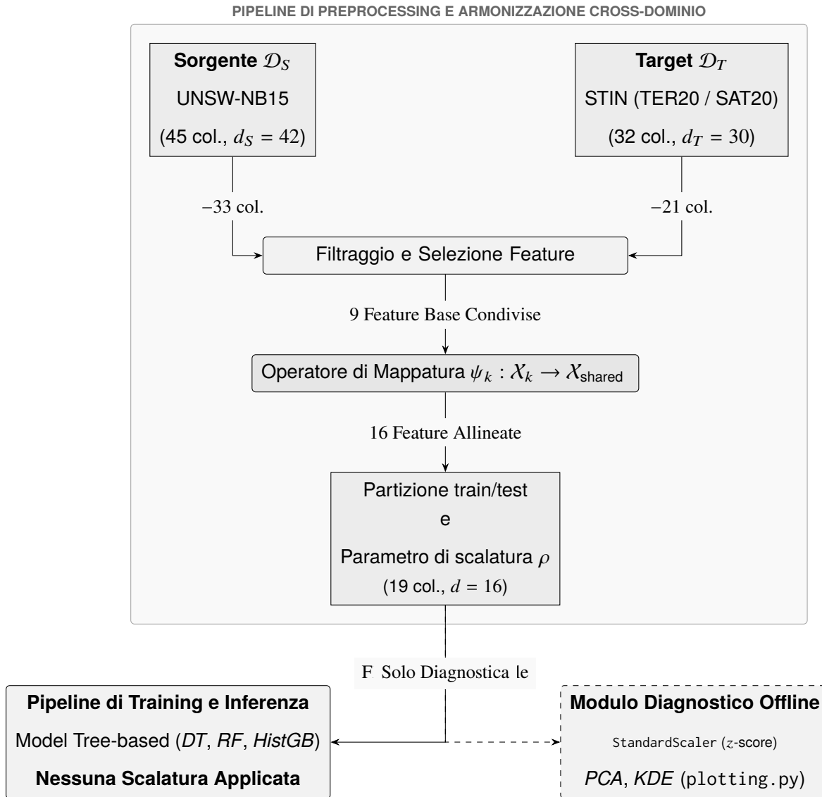
Figura 4.2: Diagramma di flusso della pipeline di preprocessing e armonizzazione tra il dominio sorgente \mathcal{D}_S e i domini target \mathcal{D}_T , dall'estrazione delle feature grezze alla generazione dello spazio coordinato finale a 16 dimensioni.
