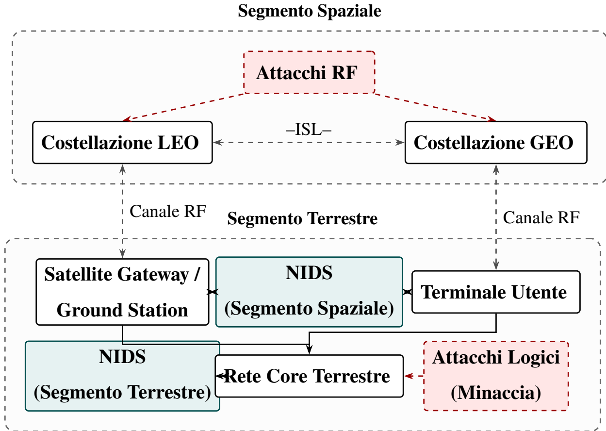
Figura 2.1: Architettura di rete integrata Terrestre-Spaziale: rappresentazione della superficie d’attacco e posizionamento dei punti di monitoraggio Network Intrusion Detection System (NIDS).
