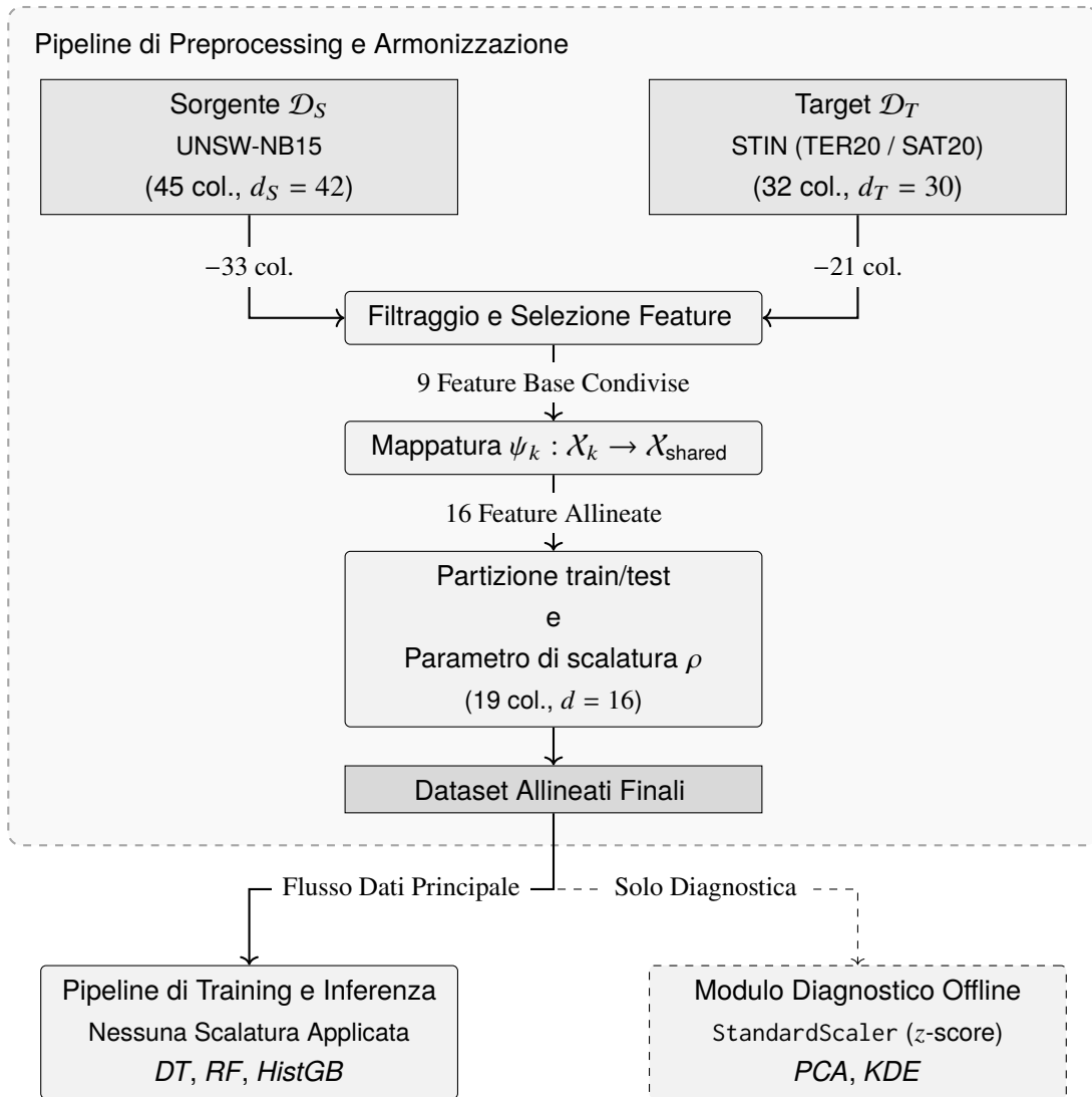
Figura 4.2: Diagramma di flusso della pipeline di preprocessing e armonizzazione tra il dominio sorgente \mathcal{D}_S e i domini target \mathcal{D}_T , dall'estrazione delle feature grezze alla generazione dello spazio coordinato finale a 16 dimensioni.
