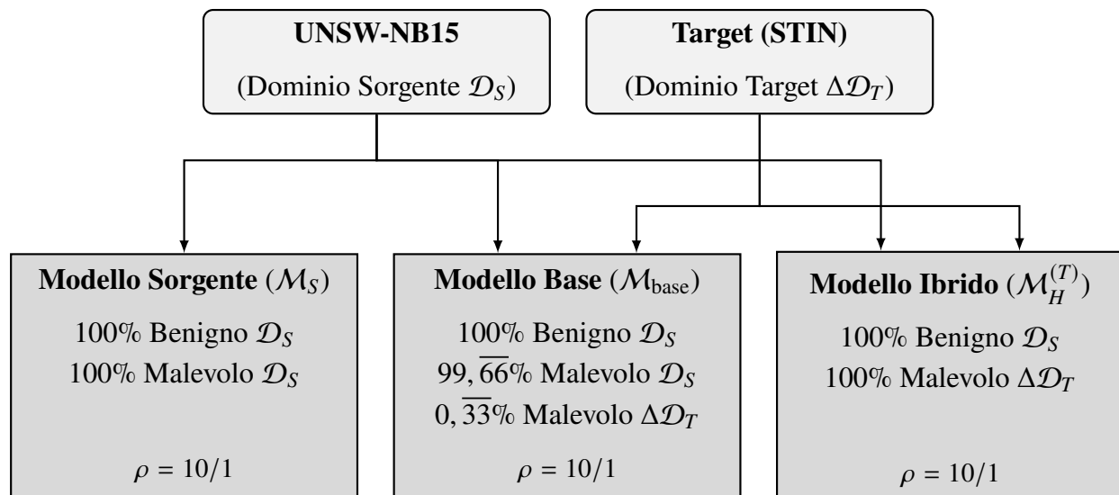
Figura 4.3: Architettura del flusso dati per l’addestramento dei Modelli Aggregati. Le percentuali indicano l’origine logica dei pacchetti che compongono i training set , forzati strutturalmente al vincolo \rho_{ben/mal} = 10/1 .
