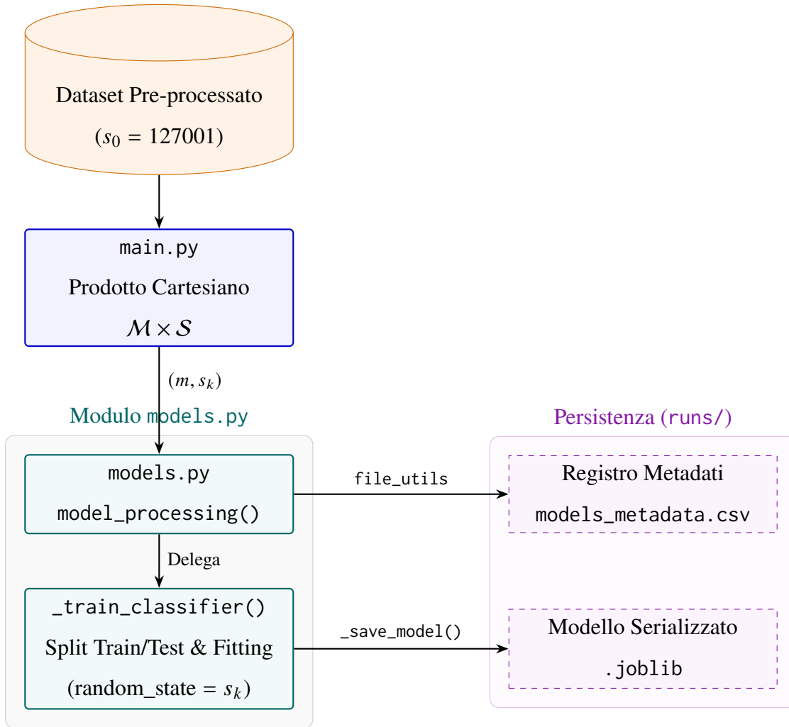
Figura 4.4: Flusso operativo dell’orchestrazione multi-seed e isolamento degli artefatti persistenti.
