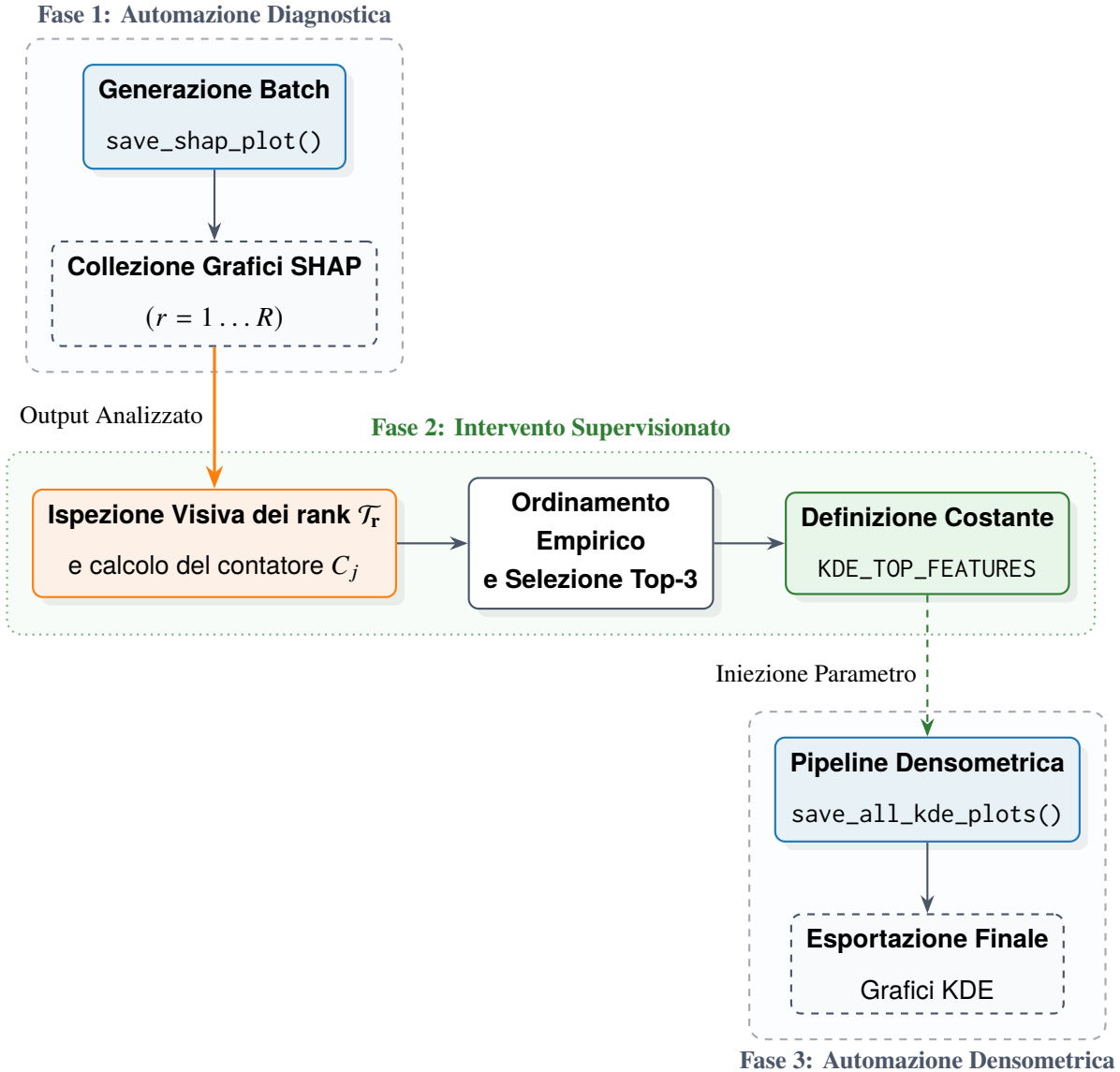
Figura 4.9: Diagramma architetturale del raccordo Human-in-the-Loop tra l'analisi diagnostica (SHAP) e la valutazione densometrica (KDE). L'intervento manuale (Fase 2) funge da disaccoppiamento metodologico tra le due pipeline automatizzate.
