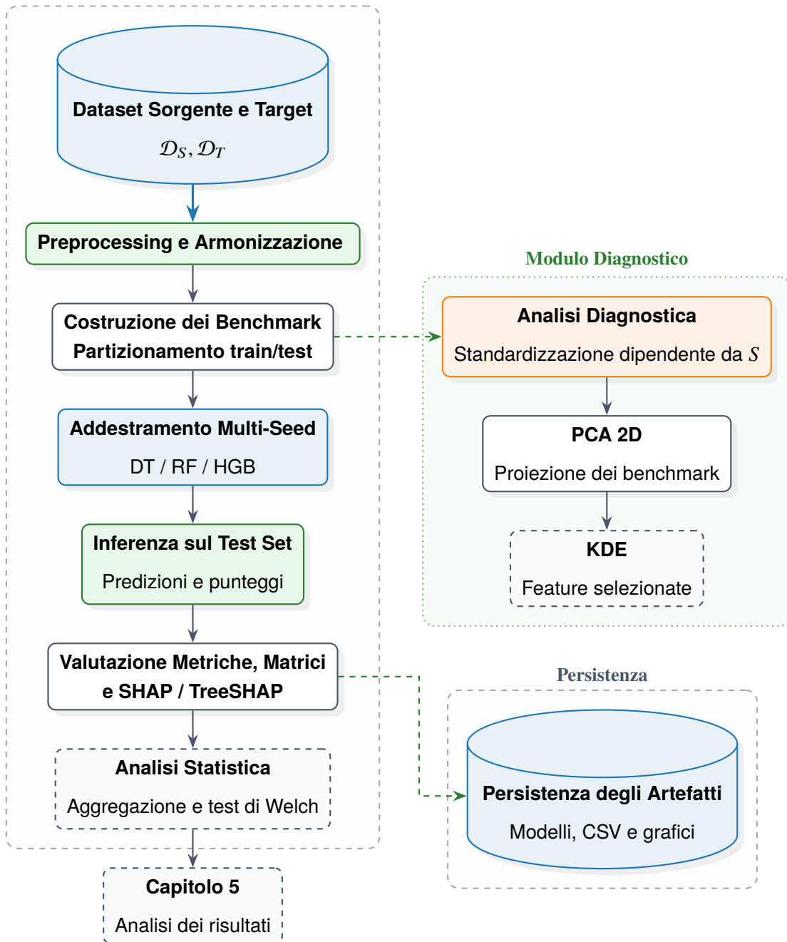
Figura 4.10: Sintesi end-to-end della pipeline implementativa. Il flusso principale attraversa le fasi di preprocessing, costruzione dei benchmark, addestramento multi-seed, inferenza, valutazione e analisi statistica; in parallelo, il modulo diagnostico realizza le procedure PCA e KDE. Gli artefatti prodotti vengono persistiti e costituiscono l'input documentale per la successiva analisi dei risultati.
