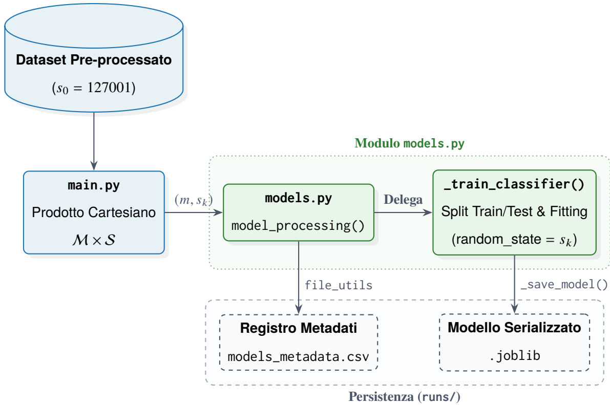
Figura 4.4: Flusso operativo dell’orchestrazione multi-seed e isolamento degli artefatti persistiti.
