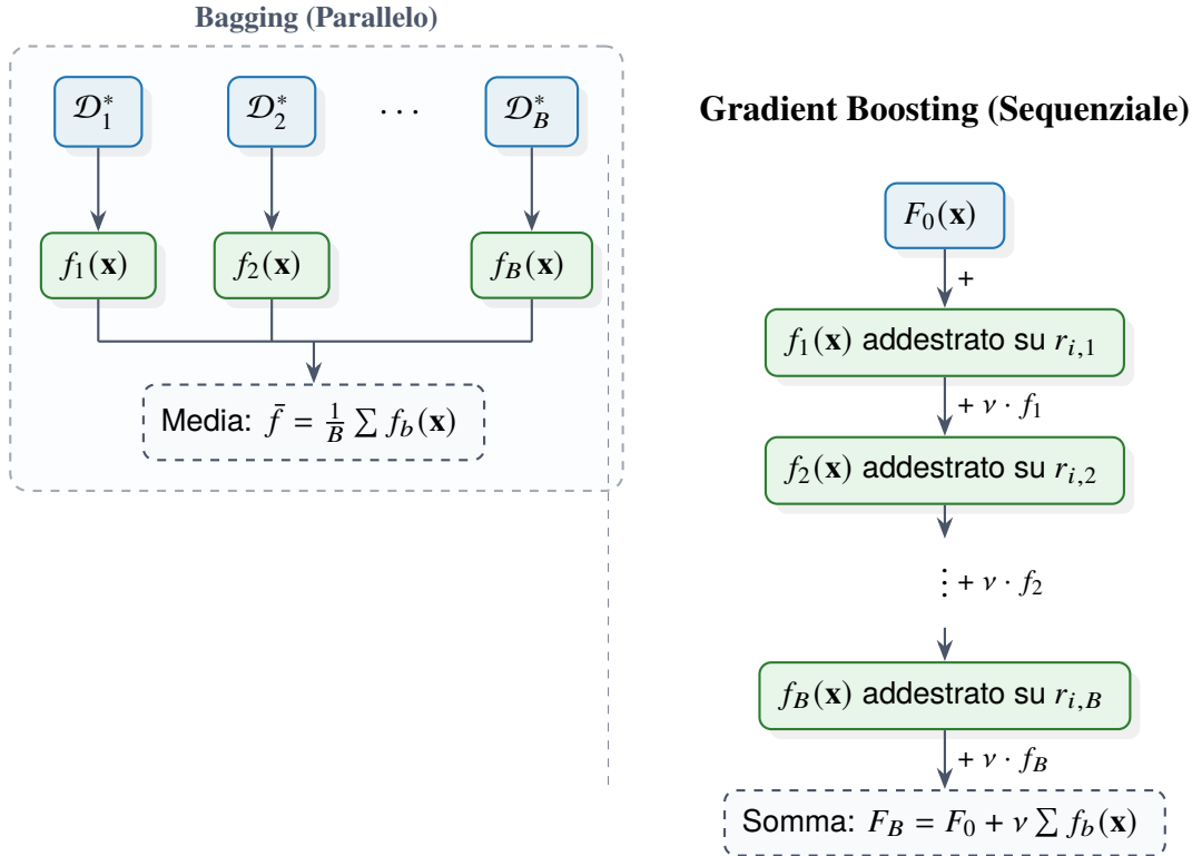
Figura 3.5: Confronto logico-procedurale tra gli schemi di aggregazione. A sinistra, il paradigma Bagging esegue un addestramento parallelo su campionamenti bootstrap indipendenti. A destra, il paradigma Gradient Boosting adotta un approccio sequenziale in cui ciascun albero mira a correggere i residui iterativi generati dall'insieme precedente.
