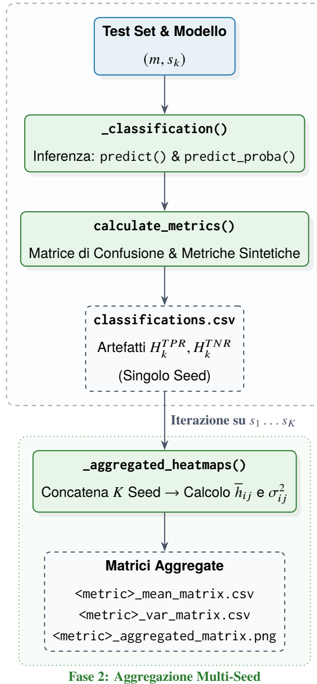
Figura 4.5: Pipeline a due stadi per il calcolo delle metriche di classificazione, tracciamento su file system e aggregazione statistica multi-seed.
