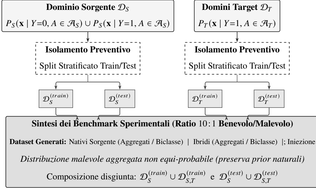
Figura 3.1: Pipeline metodologica astratta: isolamento preventivo delle partizioni per la prevenzione del data leakage , vincoli di proporzionamento 10 : 1 e sintesi delle cinque tipologie di benchmark.
