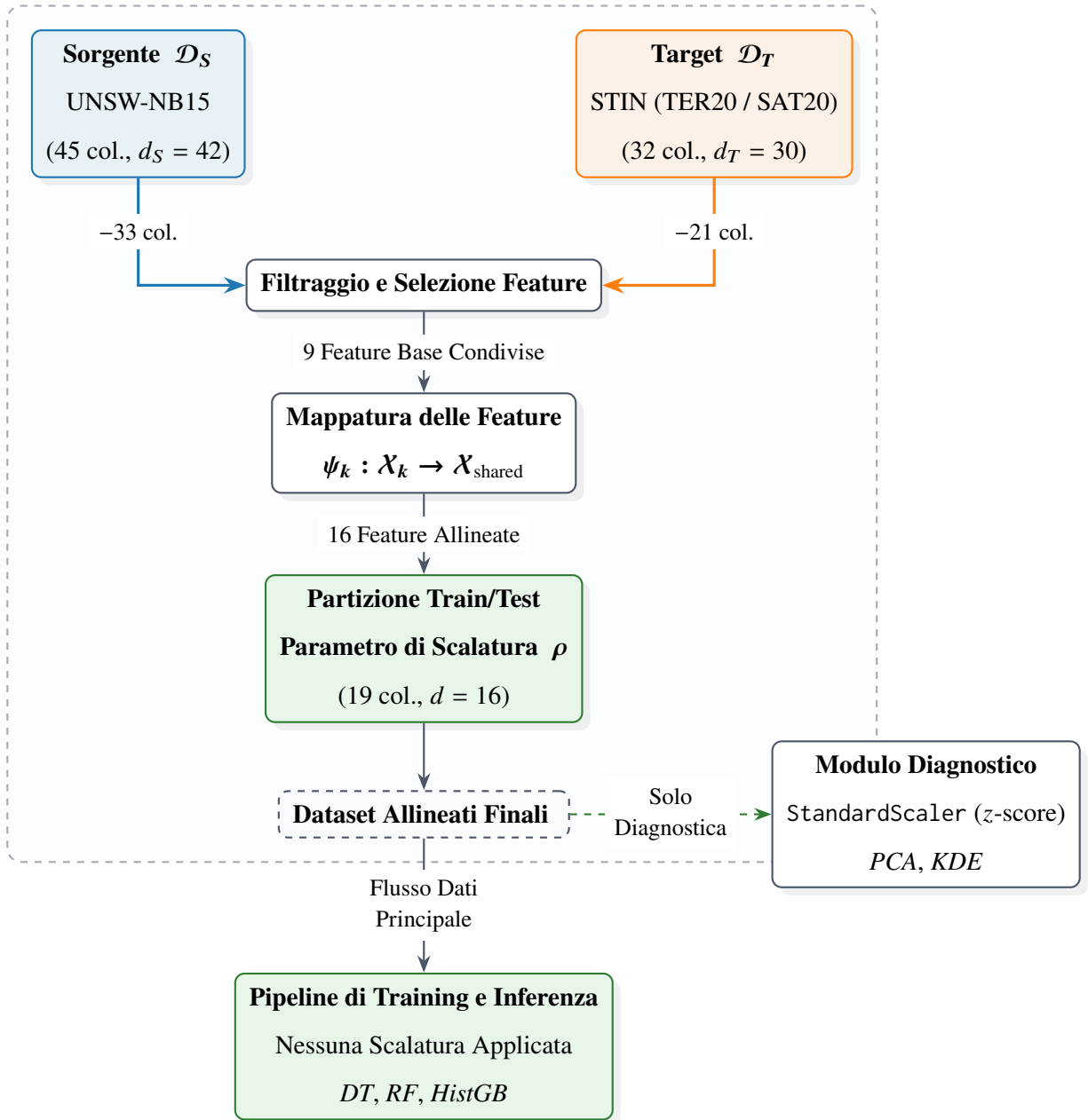
Figura 4.2: Diagramma di flusso della pipeline di preprocessing e armonizzazione tra il dominio sorgente \mathcal{D}_S e i domini target \mathcal{D}_T , dall'estrazione delle feature grezze alla generazione dello spazio coordinato finale a 16 dimensioni.
