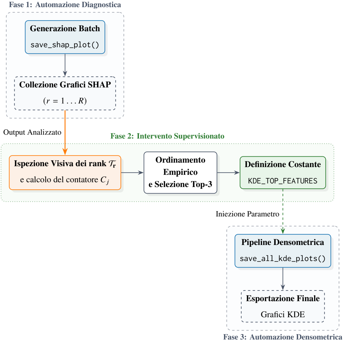
Figura 4.9: Diagramma architetturale del raccordo Human-in-the-Loop tra l'analisi diagnostica (SHAP) e la valutazione densometrica (KDE). L'intervento manuale (Fase 2) funge da disaccoppiamento metodologico tra le due pipeline automatizzate.
