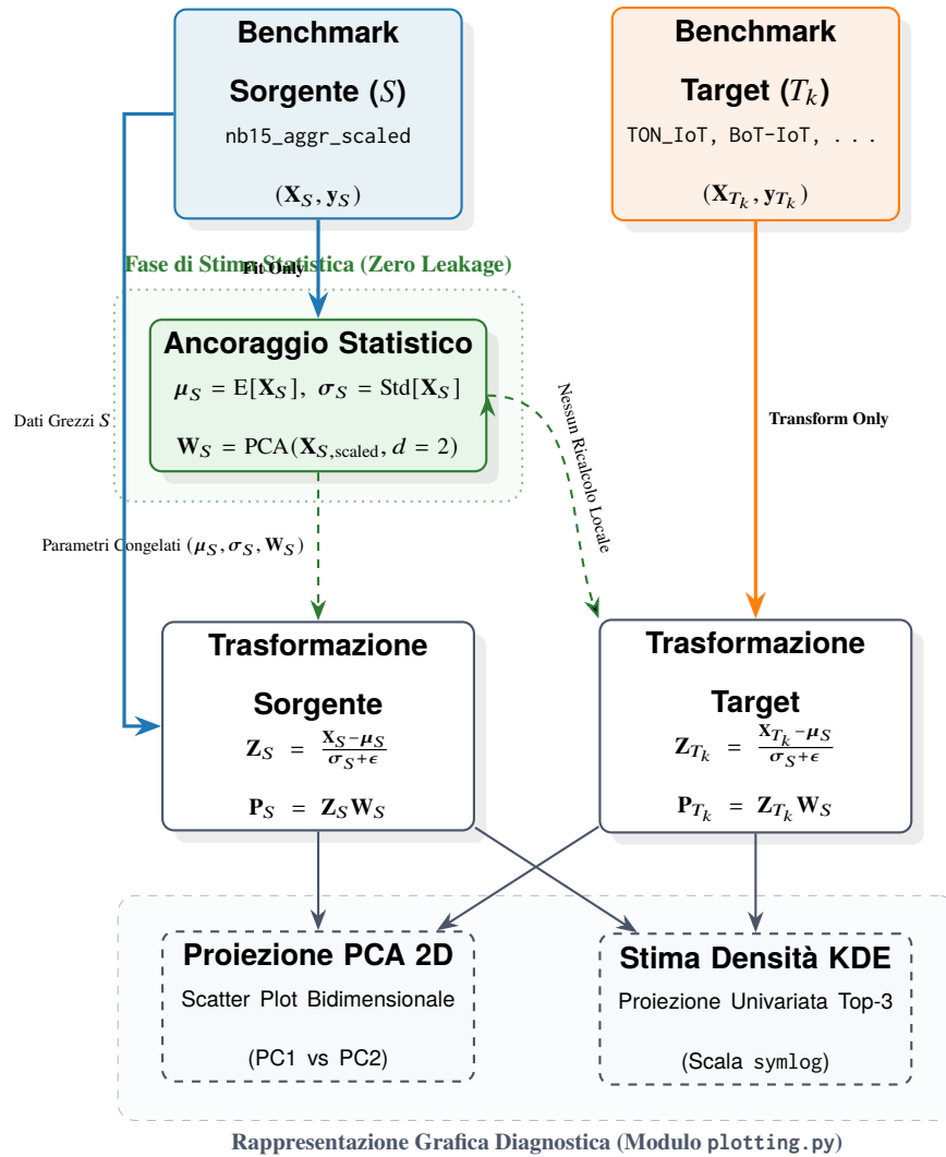
Figura 4.7: Schema concettuale della Standardizzazione Diagnostica Dipendente dal Sorgente: le statistiche di centralità e variabilità ( \mu_S, \sigma_S ) e gli autovettori della PCA ( \mathbf{W}_S ) vengono stimati esclusivamente sul benchmark sorgente S e congelati. La trasformazione dei benchmark target T_k avviene per applicazione diretta di tali parametri, preservando lo scostamento distributivo reale ( domain shift ).
