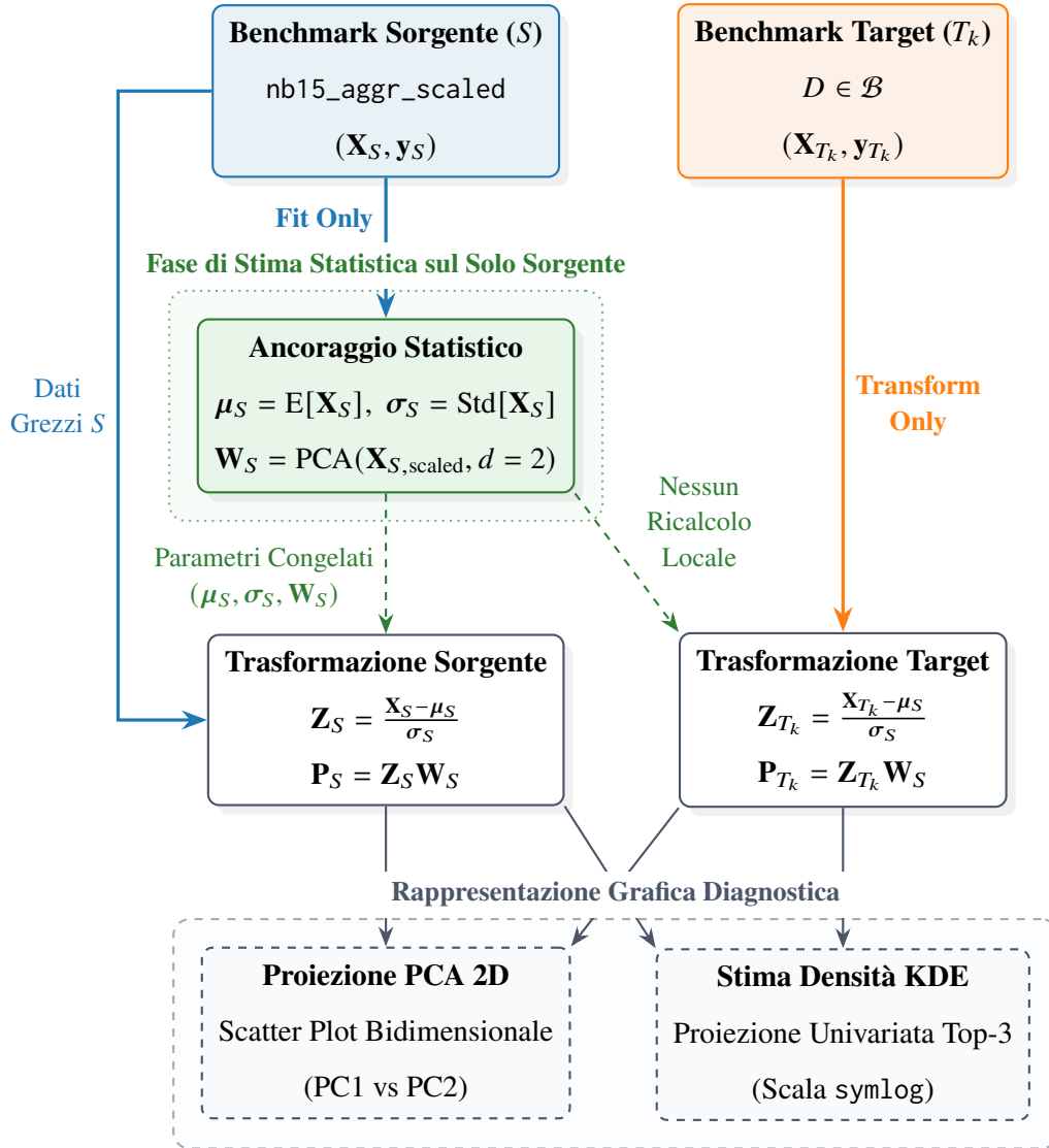
Figura 4.8: Schema concettuale della Standardizzazione Diagnostica Dipendente dal Sorgente: le statistiche di centralità e variabilità (\mu_S, \sigma_S) e gli autovettori della PCA ( \mathbf{W}_S ) vengono stimati esclusivamente sul benchmark sorgente S e congelati. La trasformazione dei benchmark target T_k avviene per applicazione diretta di tali parametri, preservando lo scostamento distributivo reale ( domain shift ).
