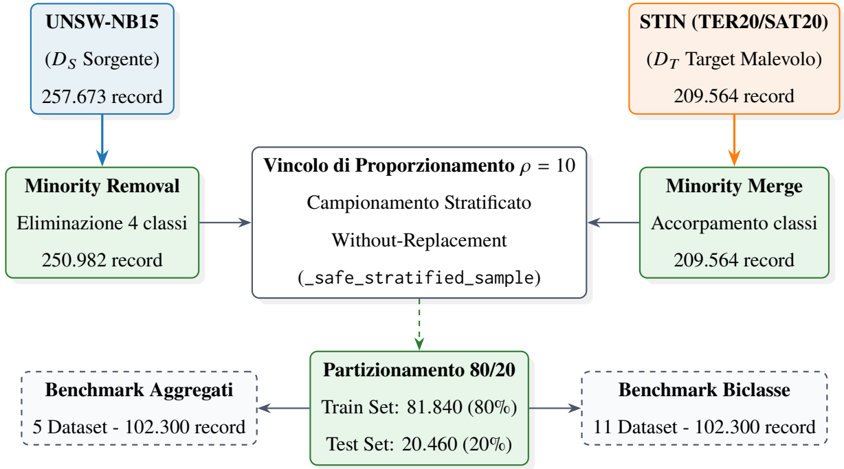
Figura 4.2: Diagramma di flusso del processo di estrazione, pulizia, campionamento vincolato ( \rho = 10 ) e partizionamento stratificato 80/20 per la generazione dei benchmark fisici aggregati e biclasse.
