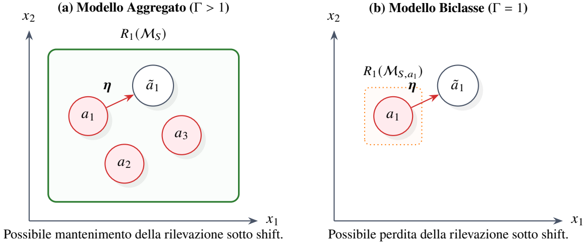
Figura 3.7: Rappresentazione concettuale, non vincolante, di possibili configurazioni della regione decisionale positiva al variare della granularità della conoscenza malevola. La figura illustra due esiti qualitativi compatibili con un domain shift , senza postulare una relazione geometrica garantita tra \Gamma(M) e la capacità di generalizzazione.
