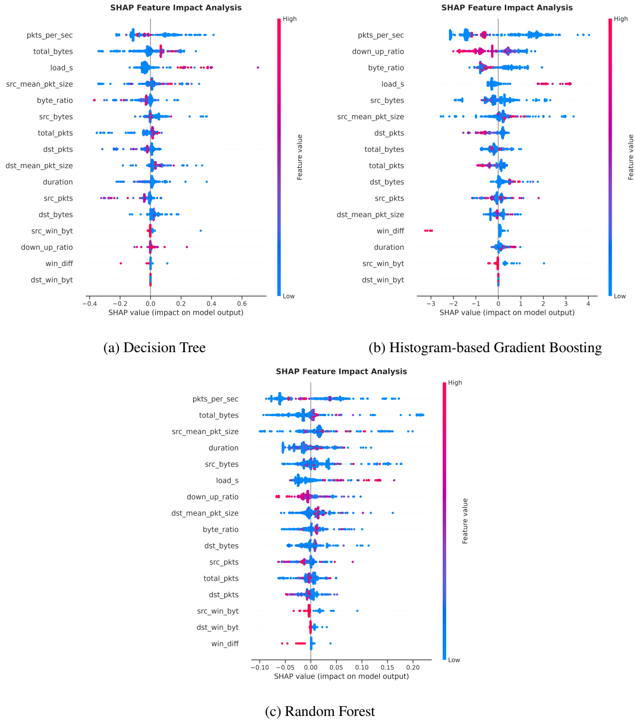
Figura 5.8: Summary plot SHAP del modello aggregato sorgente NB15 implementato mediante Decision Tree, Histogram-based Gradient Boosting e Random Forest, valutati sul test set aggregato NB15 con seed s = 42 .
