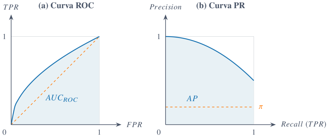
Figura 3.9: Rappresentazione schematica delle curve ROC (a) e Precision–Recall (b). L’area è illustrativa; la sintesi numerica della curva PR impiegata nella pipeline è l’Average Precision (AP).
