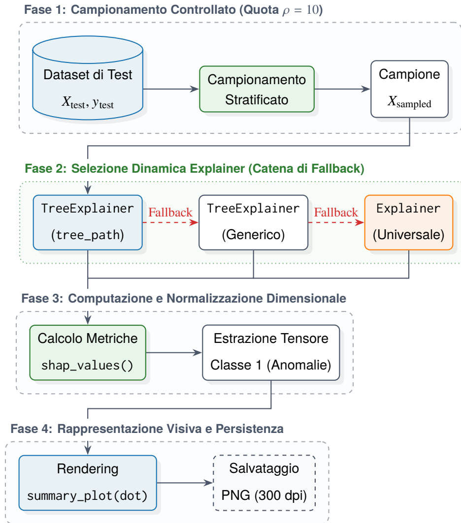
Figura 4.8: Architettura della pipeline di spiegabilità SHAP per i modelli di classificazione. Il diagramma illustra le quattro fasi sequenziali: campionamento stratificato per il contenimento computazionale, selezione con fallback del motore di spiegazione, estrazione normalizzata della componente anomala e salvataggio degli artefatti visivi.
