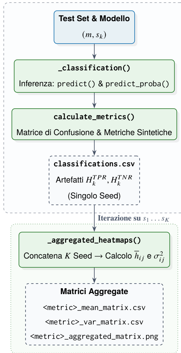
Figura 4.5: Pipeline a due stadi per il calcolo delle metriche di classificazione, tracciamento su file system e aggregazione statistica multi-seed.
