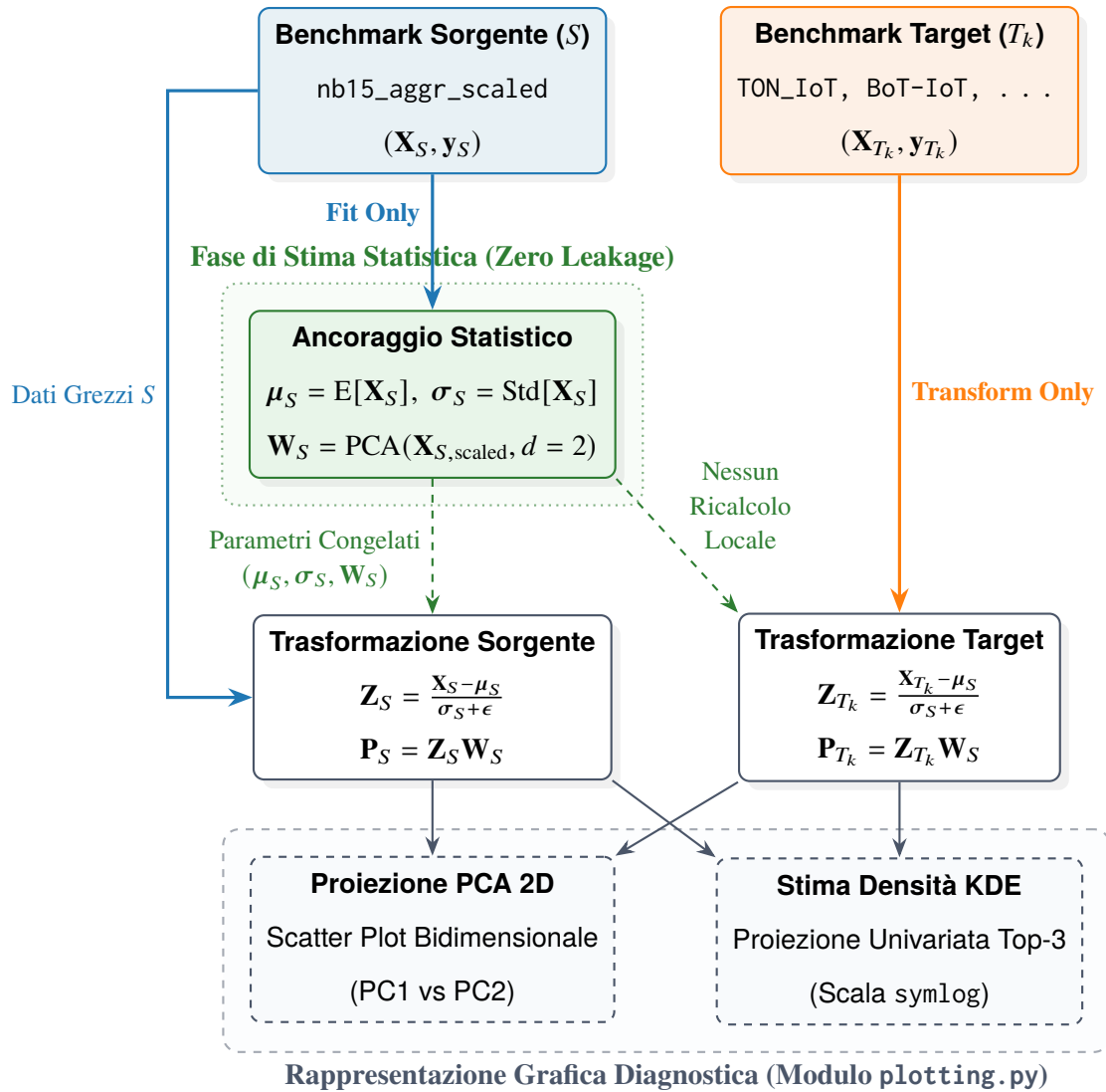
Figura 4.7: Schema concettuale della Standardizzazione Diagnostica Dipendente dal Sorgente: le statistiche di centralità e variabilità ( \mu_S, \sigma_S ) e gli autovettori della PCA ( \mathbf{W}_S ) vengono stimati esclusivamente sul benchmark sorgente S e congelati. La trasformazione dei benchmark target T_k avviene per applicazione diretta di tali parametri, preservando lo scostamento distributivo reale ( domain shift ).
