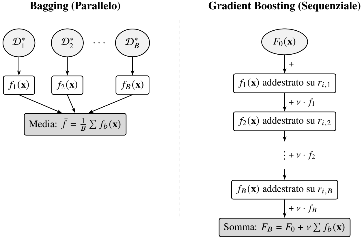
Figura 3.5: Confronto logico-procedurale tra gli schemi di aggregazione. A sinistra, il paradigma Bagging esegue un addestramento parallelo su campionamenti bootstrap indipendenti. A destra, il paradigma Gradient Boosting adotta un approccio sequenziale in cui ciascun albero mira a correggere i residui iterativi generati dall'insieme precedente.
