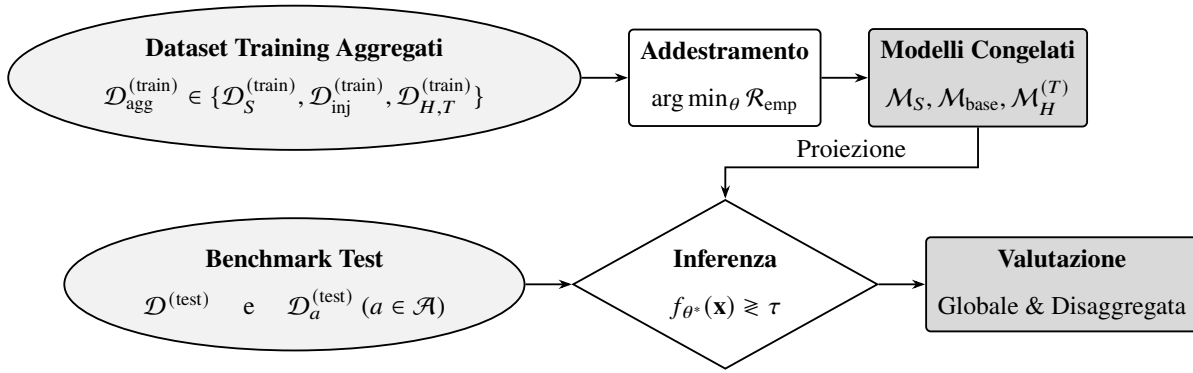
Figura 3.3: Flusso concettuale del protocollo di addestramento, inferenza e disaggregazione delle prestazioni per i modelli aggregati ( \mathcal{M}_{\text{base}}, \mathcal{M}_S, \mathcal{M}_H^{(T)} ). I modelli, congelati post-ottimizzazione, vengono valutati sia sull'intero benchmark multi-classe per misurare la generalizzazione di dominio, sia sulle singole partizioni per famiglia d'attacco \mathcal{D}_a^{(\text{test})} per l'analisi di disaggregazione puntuale.
