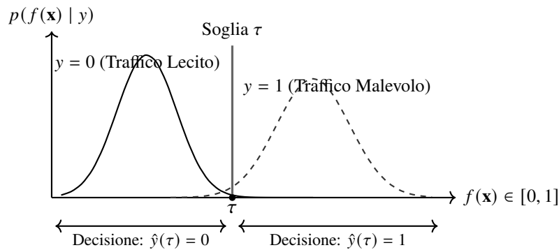
Figura 3.8: Mappatura della probabilità a posteriori f(\mathbf{x}) sulla regola decisionale binaria \hat{y}(\tau) in funzione della soglia \tau .
