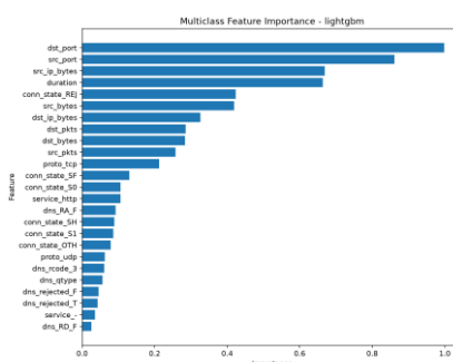
Figura 14 - Importanza delle feature nel modello LightGBM multiclasse
