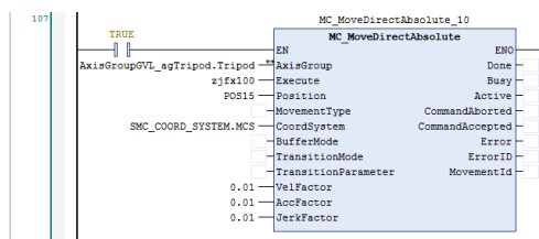
图 7 PLC 程序：Delta 机器人移开进行拍照
