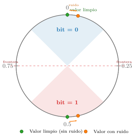
Figura 5.14: Codificación en el toro \mathbb{T} = \mathbb{R}/\mathbb{Z} . El bit 0 se codifica cerca de 0.0 (arriba) y el bit 1 cerca de 0.5 (abajo). El ruido desplaza la posición, pero el bit se recupera mientras no cruce la frontera de decisión.
