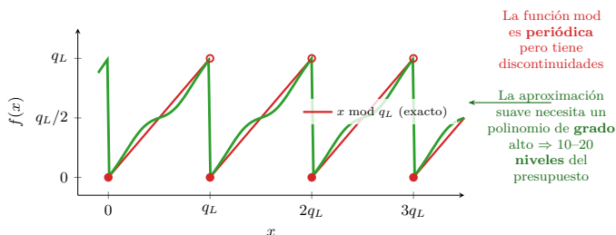
Figura 5.8: Aproximación de la reducción modular. La función « x módulo q_L » es periódica pero discontinua — no se puede expresar como una secuencia de sumas y multiplicaciones. Para evaluarla homomórficamente se aproxima mediante un polinomio de grado alto, que consume entre 10 y 20 niveles multiplicativos.
