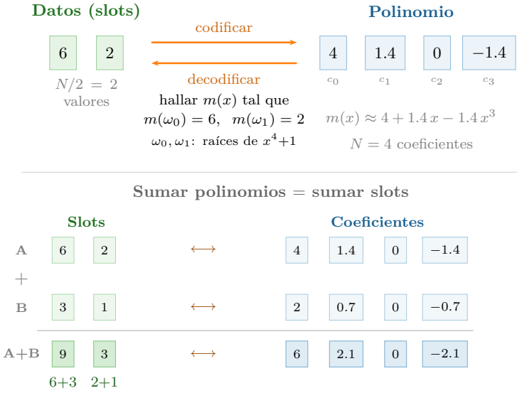
Figura 5.11: Codificación por slots ( N = 4 ). Arriba: dos datos [6, 2] se codifican como un polinomio de 4 coeficientes hallando m(x) tal que m(\omega_0) = 6 y m(\omega_1) = 2 . Abajo: sumar dos polinomios coeficiente a coeficiente equivale a sumar los slots dato a dato — la base del paralelismo SIMD.
