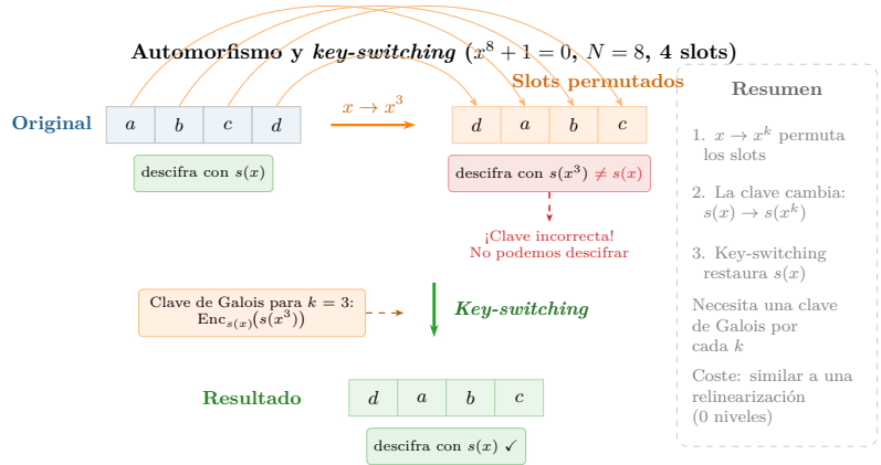
Figura 5.13: Automorfismo y key-switching (ejemplo con x^8 + 1 = 0 , N = 8 , 4 slots). La sustitución x \rightarrow x^3 permuta cíclicamente los slots: [a, b, c, d] \rightarrow [d, a, b, c] . Pero cambia la clave de descifrado de s(x) a s(x^3) . El key-switching, usando una clave de Galois precalculada, restaura la clave original sin revelar el secreto.
