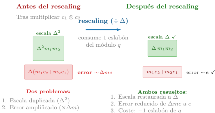
Figura 5.6: Rescaling: dividir por \Delta corrige simultáneamente la escala duplicada y el error amplificado, a cambio de consumir un eslabón de la cadena de módulos.
