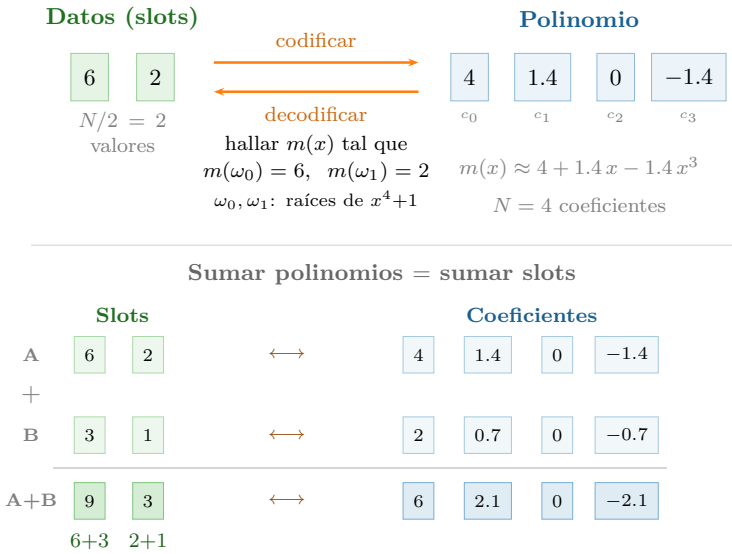
Figura 5.11: Codificación por slots ( N = 4 ). Arriba: dos datos [6, 2] se codifican como un polinomio de 4 coeficientes hallando m(x) tal que m(\omega_0) = 6 y m(\omega_1) = 2 . Abajo: sumar dos polinomios coeficiente a coeficiente equivale a sumar los slots dato a dato — la base del paralelismo SIMD.
