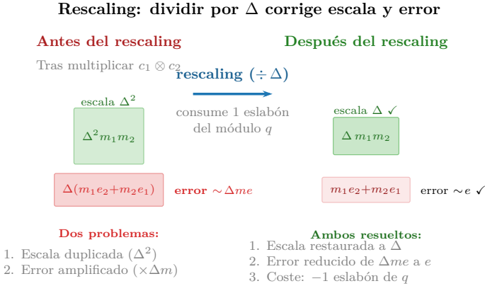
Figura 5.6: Rescaling: dividir por \Delta corrige simultáneamente la escala duplicada y el error amplificado, a cambio de consumir un eslabón de la cadena de módulos.
