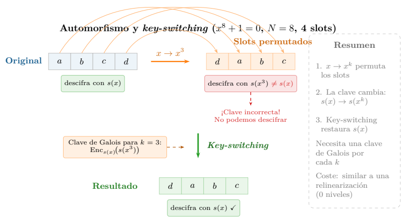
Figura 5.13: Automorfismo y key-switching (ejemplo con x^8 + 1 = 0 , N = 8 , 4 slots). La sustitución x \rightarrow x^3 permuta cíclicamente los slots: [a, b, c, d] \rightarrow [d, a, b, c] . Pero cambia la clave de descifrado de s(x) a s(x^3) . El key-switching, usando una clave de Galois precalculada, restaura la clave original sin revelar el secreto.
