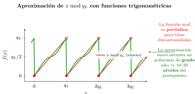
Figura 5.8: Aproximación de la reducción modular. La función « x módulo q_L » es periódica pero discontinua — no se puede expresar como una secuencia de sumas y multiplicaciones. Para evaluarla homomórficamente se aproxima mediante un polinomio de grado alto, que consume entre 10 y 20 niveles multiplicativos.
