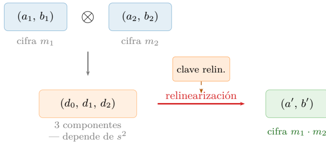
Figura 5.5: Multiplicación entre cifrotextos. El producto genera un triplete (d_0, d_1, d_2) que depende de s^2 . La relinearización, usando una clave pública que cifra s^2 , lo reduce a un par estándar (a', b') descifable con s .
