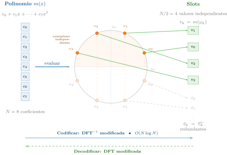
Figura 5.10: Inmersión canónica. Los coeficientes del polinomio m(x) no son los datos: los slots son las evaluaciones de m(x) en las N raíces complejas de x^N + 1 . Las raíces conjugadas producen valores redundantes, dejando N/2 slots independientes. Codificar y decodificar equivale a una DFT modificada (inversa y directa, respectivamente).
