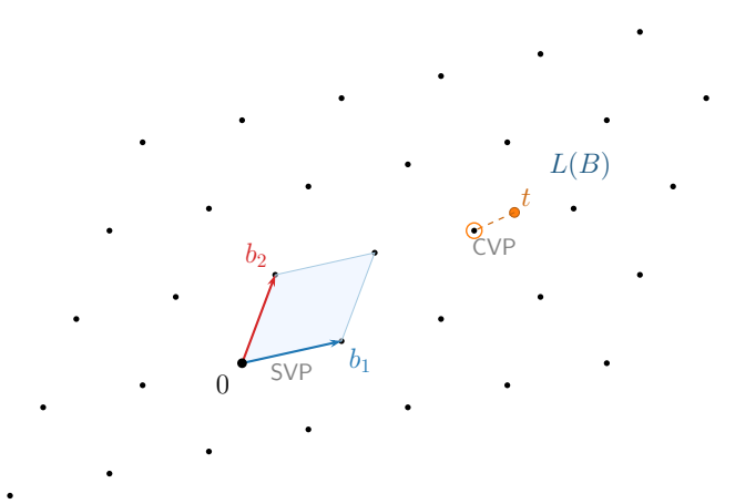
Figura 5.1: Retículo bidimensional generado por dos vectores base b_1 y b_2 . La región sombreada es el dominio fundamental (paralelogramo definido por la base). El punto t está fuera del retículo: encontrar el punto del retículo más cercano (CVP) o el vector no nulo más corto (SVP) es computacionalmente intratable en dimensiones altas.
