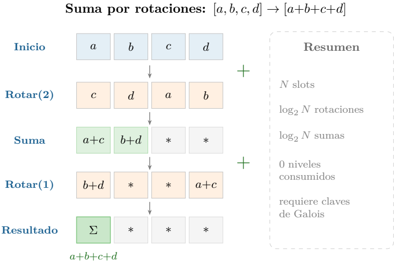
Figura 5.12: Suma por rotaciones. Con 4 slots, dos pasos de rotar-y-sumar bastan para acumular la suma total en el primer slot. El diagrama muestra la vista por slots; internamente, cada «Suma» es una adición de los N coeficientes de dos polinomios, que por linealidad de la evaluación produce la suma slot a slot. Las rotaciones requieren claves de Galois, pero no consumen niveles multiplicativos.
