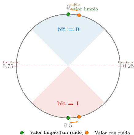
Figura 5.14: Codificación en el toro \mathbb{T} = \mathbb{R}/\mathbb{Z} . El bit 0 se codifica cerca de 0.0 (arriba) y el bit 1 cerca de 0.5 (abajo). El ruido desplaza la posición, pero el bit se recupera mientras no cruce la frontera de decisión.
