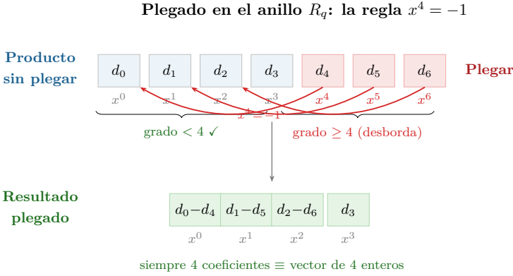
Figura 5.2: Plegado en el anillo R_q . Al multiplicar polinomios, los términos de grado mayor o igual que n se pliegan al rango [0, n - 1] mediante la regla x^n = -1 . Esta restricción equivale a trabajar con matrices anticirculantes, codificando una matriz de n \times n enteros en solo n coeficientes.
