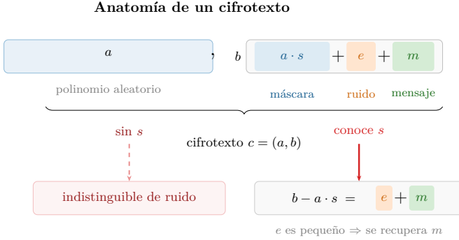
Figura 5.4: Anatomía de un cifrotexto. El par (a, b) contiene el mensaje m oculto tras una máscara a \cdot s y un ruido e . Quien conoce s elimina la máscara y recupera m ; sin s , el cifrotexto es indistinguible de ruido aleatorio.
