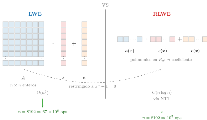
Figura 5.3: LWE frente a RLWE. A la izquierda, LWE requiere una matriz A de n \times n enteros. A la derecha, RLWE codifica la misma información en un polinomio de n coeficientes, reduciendo el coste de O(n^2) a O(n \log n) vía la NTT.
