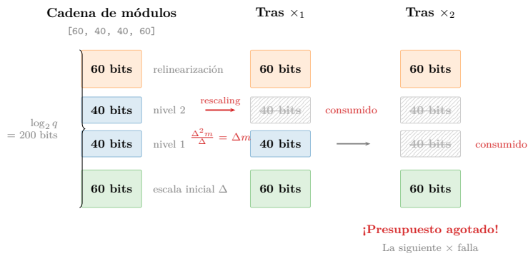
Figura 5.7: Cadena de módulos y consumo de niveles. Cada multiplicación consume un eslabón de 40 bits mediante rescaling. Cuando se agotan los eslabones intermedios, la siguiente multiplicación falla.
