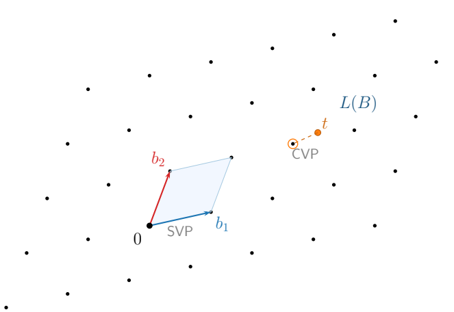
Figura 5.1: Retículo bidimensional generado por dos vectores base b_1 y b_2 . La región sombreada es el dominio fundamental (paralelogramo definido por la base). El punto t está fuera del retículo: encontrar el punto del retículo más cercano (CVP) o el vector no nulo más corto (SVP) es computacionalmente intratable en dimensiones altas.
