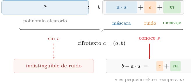
Figura 5.4: Anatomía de un cifrotexto. El par (a, b) contiene el mensaje m oculto tras una máscara a \cdot s y un ruido e . Quien conoce s elimina la máscara y recupera m ; sin s , el cifrotexto es indistinguible de ruido aleatorio.
