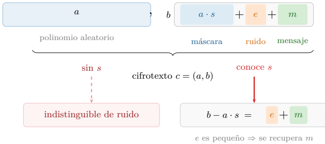
Figura 5.4: Anatomía de un cifrotexto. El par (a, b) contiene el mensaje m oculto tras una máscara a \cdot s y un ruido e . Quien conoce s elimina la máscara y recupera m ; sin s , el cifrotexto es indistinguible de ruido aleatorio.
