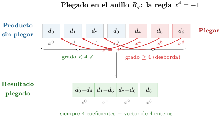
Figura 5.2: Plegado en el anillo R_q . Al multiplicar polinomios, los términos de grado mayor o igual que N se pliegan al rango [0, N-1] mediante la regla x^N = -1 . Esta restricción equivale a trabajar con matrices anticirculantes, codificando una matriz de N \times N enteros en solo N coeficientes.
