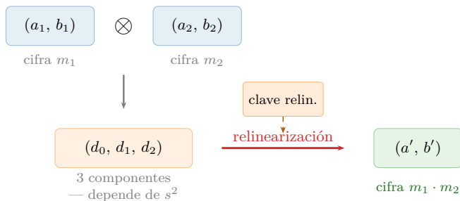
Figura 5.5: Multiplicación entre cifrotextos. El producto genera un triplete (d_0, d_1, d_2) que depende de s^2 . La relinearización, usando una clave pública que cifra s^2 , lo reduce a un par estándar (a', b') descifrable con s .
