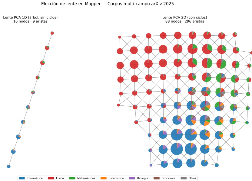
Figura 2.10: Comparación de lentes Mapper sobre el corpus arXiv 2025 (8.085 artículos). Izquierda: lente PCA 1D — árbol de 10 nodos y 9 aristas, sin ciclos. Derecha: lente PCA 2D — red de 88 nodos y 296 aristas con ciclos interdisciplinares. La misma paleta de colores que en la Figura 2.11.
