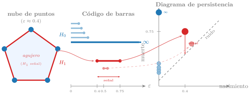
Figura 5.4: Izquierda: cinco puntos dispuestos en un pentágono regular a escala \varepsilon \approx 0.4 — las aristas (rojo) forman un bucle cerrado y el interior sombreado es el agujero que origina la característica H_1 . Centro: código de barras de la nube; las cuatro barras azules cortas son H_0 de ruido (componentes que se fusionan rápido), la barra azul larga con flecha es el H_0 inmortal, la barra roja larga es la señal H_1 (el agujero) y la barra roja muy corta es ruido H_1 . Derecha: diagrama de persistencia; los puntos azules pequeños cerca de la diagonal son ruido H_0 , el punto rojo grande alejado de la diagonal es la señal H_1 , y el punto rojo pequeño junto a la diagonal es el ruido H_1 . La distancia al eje diagonal mide la persistencia: señal arriba, ruido abajo. Las flechas muestran la correspondencia barra — punto.
