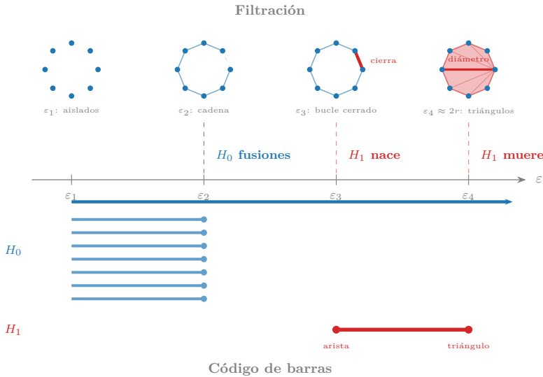
Figura 5.3: Cuatro fotografías de la filtración sincronizadas con el código de barras. \varepsilon_2 : las aristas forman una cadena ( \beta_0 = 1 , \beta_1 = 0 ). \varepsilon_3 : la arista roja cierra el bucle — H_1 nace ( \beta_1 = 1 ). \varepsilon_4 : cuando \varepsilon alcanza el diámetro ( 2r ), los triángulos en abanico —formados solo por puntos del anillo, sin punto central— rellenan el interior y H_1 muere ( \beta_1 = 0 ). El diámetro (línea roja gruesa) es la cuerda crítica.
