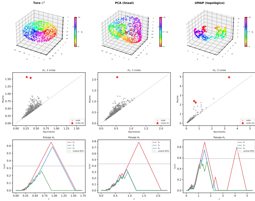
Figura 2.12: Receta 7: reducción de un toro ( \beta_1 = 2 ) desde \mathbb{R}^{50} a \mathbb{R}^3 con PCA (columna central) y UMAP (columna derecha), con el toro original en \mathbb{R}^3 como referencia (columna izquierda). Fila superior: nubes 3D coloreadas por \theta — PCA puede parecer geoméricamente limpia, UMAP suele verse distorsionada: ambas apariencias son engañosas. Fila central: diagrama de persistencia H_1 , estrellas rojas = ciclos persistentes; PCA detecta 1, UMAP detecta 2. Fila inferior: paisaje de persistencia con capas \lambda_1 (rojo) y \lambda_2 (azul), umbral nulo al 95% (línea discontinua) — solo UMAP tiene ambas capas sobre el umbral, confirmando \beta_1 = 2 .
