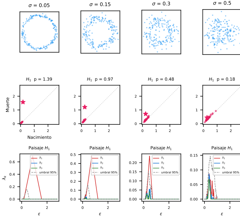
Figura 2.5: Receta 3 — estabilidad: arriba, el mismo círculo con cuatro niveles de ruido creciente ( \sigma ); centro, diagrama de persistencia H_1 (la estrella marca el agujero principal); abajo, paisaje de persistencia \lambda_1 con el umbral 95%. La señal decrece gradualmente — nunca desaparece de golpe.
