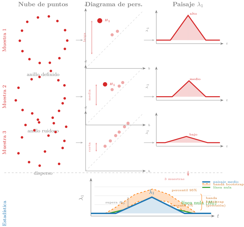
Figura 5.7: Tres muestras del mismo proceso (filas 1–3) producen diagramas de persistencia con barras de distinta longitud y paisajes con picos de distinta altura. La fila inferior superpone los tres paisajes individuales (rojo) para obtener el paisaje medio (azul), la banda bootstrap 5%–95% (naranja, banda de variabilidad de remuestras del dataset original) y la línea nula (verde, percentil 95% de paisajes de datos permutados). El pico azul supera la línea nula — señal estadísticamente significativa — y queda dentro de la banda bootstrap — señal reproducible.
