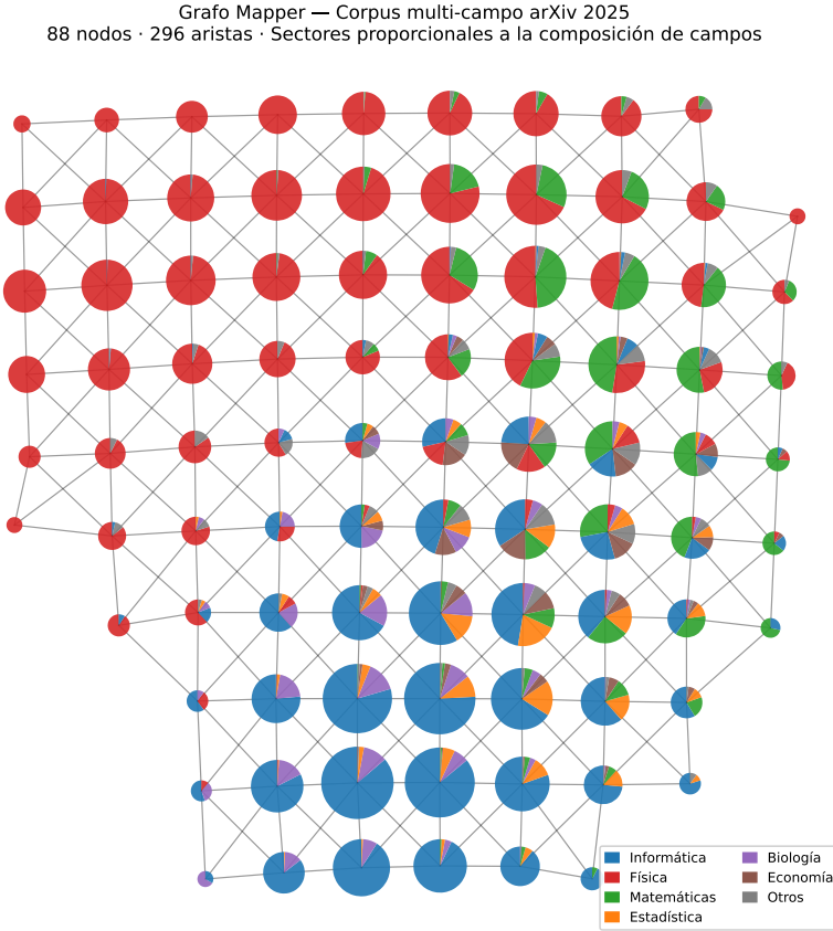
Figura 2.11: Grafo Mapper del corpus multi-campo arXiv 2025 (8.085 artículos, 88 nodos, lente PCA 2D). Cada nodo se dibuja como un pastel de sectores proporcionales a la composición de campos (azul = Informática, rojo = Física, verde = Matemáticas, naranja = Estadística, violeta = Biología, marrón = Economía). El tamaño es proporcional al número de papers. Los nodos de un único color son monodisciplinares; los de varios colores son puentes interdisciplinares.
