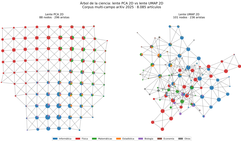
Figura 2.14: Receta 8 (árbol de la ciencia): comparación de lentes Mapper sobre el corpus arXiv 2025. Izquierda: lente PCA 2D con clustering PCA 20D — 88 nodos y 296 aristas. Derecha: lente UMAP 2D con DBSCAN coseno sobre \mathbb{R}^{384} — 101 nodos y 236 aristas. Con UMAP, las disciplinas se agrupan geográficamente según la variedad no lineal del corpus: los campos con vocabulario más similar aparecen contiguos, y los nodos multicolor (puentes interdisciplinarios) se concentran en las zonas de transición.
