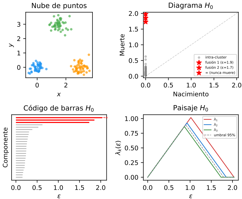
Figura 2.1: Receta 1: tres clusters gaussianos y tres representaciones equivalentes de su homología H_0 . Las tres estrellas rojas en el diagrama corresponden a los 3 clusters. En el paisaje de persistencia, los picos sobrepasan claramente el umbral de hipótesis nula (línea discontinua).
