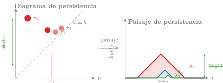
Figura 5.6: De diagrama de persistencia a paisaje. Cada punto (b_i, d_i) del PD genera una tienda de campaña \Lambda_i (panel izquierdo, coloreada por persistencia). El paisaje \lambda_k toma el k -ésimo máximo a cada escala t (panel derecho). Los niveles \lambda_1, \lambda_2, \lambda_3 capturan señal de persistencia decreciente: \lambda_1 refleja la característica dominante, \lambda_2 la secundaria.
