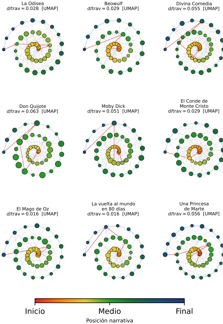
Figura 2.13: Receta 8 (camino del héroe): hipergrafo en espiral con lente UMAP 2D y DBSCAN con distancia coseno sobre los embeddings originales en \mathbb{R}^{384} . La lente no lineal organiza los parches del Mapper; los nodos se colocan en la espiral según su posición narrativa media (centro = inicio, exterior = final). Las flechas rojas (retorno) siguen cruzando casi todo el grafo, confirmando que el inicio y el final están semánticamente alejados en todas las novelas.
