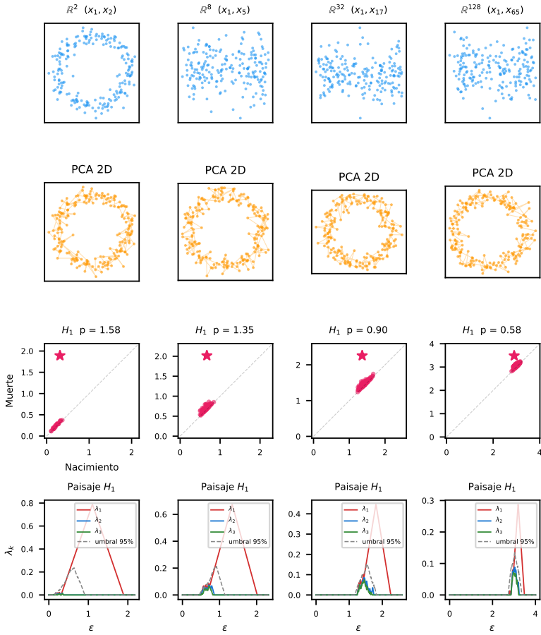
Figura 2.6: Maldición de la dimensionalidad: círculo de R = 1.5 embebido en \mathbb{R}^2 , \mathbb{R}^8 , \mathbb{R}^{32} y \mathbb{R}^{128} con ruido \sigma = 0.2 . Fila 1: proyección (x_1, x_{d/2+1}) — en alta dimensión, coordenada de ruido puro. Fila 2: PCA 2D — recupera el círculo siempre (escenario ideal para PCA). Fila 3: diagrama H_1 — la estrella más persistente se acerca a la diagonal. Fila 4: paisaje \lambda_1 — la razón señal/ruido decrece; en \mathbb{R}^{128} los picos de H_1 son difícilmente distinguibles del umbral de permutación.
