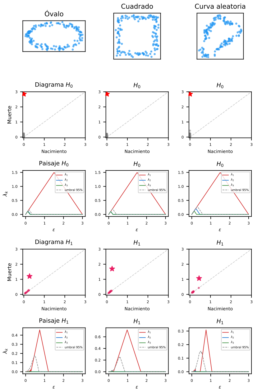
Figura 2.4: Invarianza topológica: un óvalo, un cuadrado y una curva aleatoria — tres geometrías distintas con la misma topología. En todos los casos, H_0 detecta una componente y H_1 detecta un ciclo persistente (estrella). La forma geométrica cambia; la forma topológica, no.
