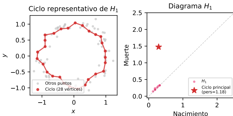
Figura 2.7: Receta 4: ciclo representativo del agujero principal. Izquierda: los vértices del ciclo (rojo) y sus aristas forman un polígono cerrado que encierra la región vacía central del anillo; los demás puntos aparecen en gris. Derecha: diagrama de persistencia H_1 con la estrella marcando la característica extraída.
