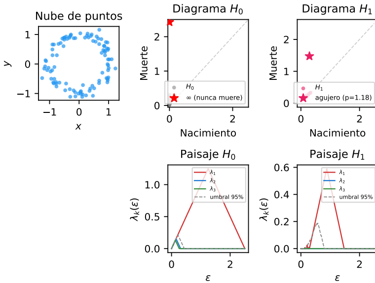
Figura 2.3: Receta 2: arriba, nube de puntos sobre un círculo con ruido, diagrama de persistencia H_0 y diagrama H_1 — la estrella rosa es el agujero central, lejos de la diagonal. Abajo, diagramas de paisajes con el umbral de hipótesis nula al 95% de confianza (línea discontinua): en H_0 , \lambda_1 sobresale (la componente inmortal) pero \lambda_2 y \lambda_3 no — hay una sola pieza; en H_1 , \lambda_1 supera claramente el umbral, confirmando que el agujero es señal.
