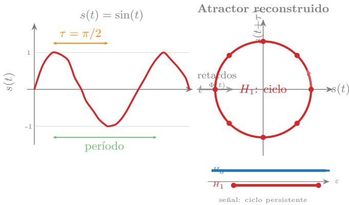
Figura 5.9: Embedding de retardos de s(t) = \sin(t) con retardo \tau = \pi/2 . Izquierda: la señal escalar s(t) vs. t . Derecha: la trayectoria (s(t), s(t+\tau)) en \mathbb{R}^2 traza un círculo limpio. El mini-barcode inferior muestra una componente inmortal en H_0 y un ciclo muy persistente en H_1 — la firma topológica de la periodicidad.
