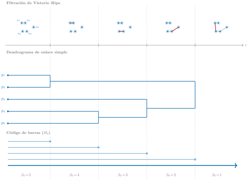
Figura 5.2: Filtración de Vietoris-Rips sobre cinco puntos (arriba), dendrograma de enlace simple (centro) y código de barras de H_0 (abajo), alineados por la misma escala \epsilon . Cada fotograma muestra la arista que provoca la fusión (en rojo); el número \beta_0 indica cuántas componentes conexas quedan activas entre eventos. La barra inmortal (flecha) es la componente que persiste para siempre.
