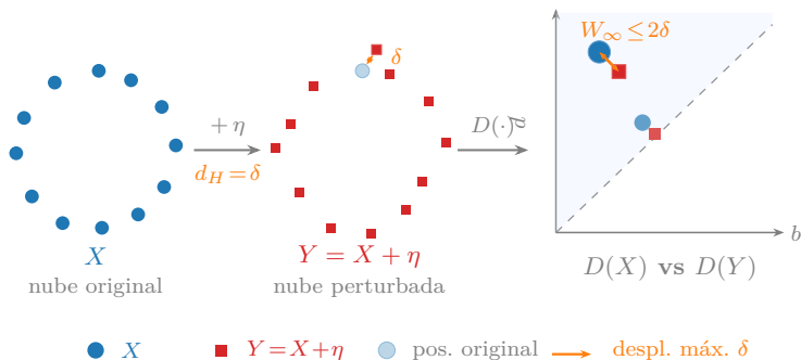
Figura 5.5: Ilustración del teorema de estabilidad en tres pasos. Izquierda: nube original X (puntos azules). Centro: nube perturbada Y = X + \eta ; el punto pálido muestra la posición original; la flecha naranja marca el peor desplazamiento \delta = d_H(X, Y) . Derecha: diagramas de persistencia D(X) (círculos) y D(Y) (cuadrados) superpuestos; las líneas grises muestran el emparejamiento bottleneck óptimo; la flecha naranja acota el mayor desplazamiento en el espacio de PDs, que no puede superar W_\infty \leq 2\delta .
