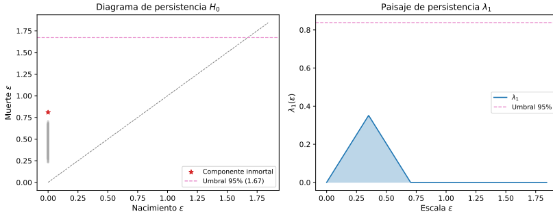
Figura 2.9: Análisis H_0 del corpus multi-campo (8.085 artículos de arXiv 2025, 29 categorías). Izquierda: diagrama de persistencia — todos los puntos cerca de la diagonal, ninguna barra supera el umbral del 95%. Derecha: paisaje \lambda_1 con umbral nulo (línea discontinua). La ciencia arXiv es una única componente conexa a nivel de significación estadística.
