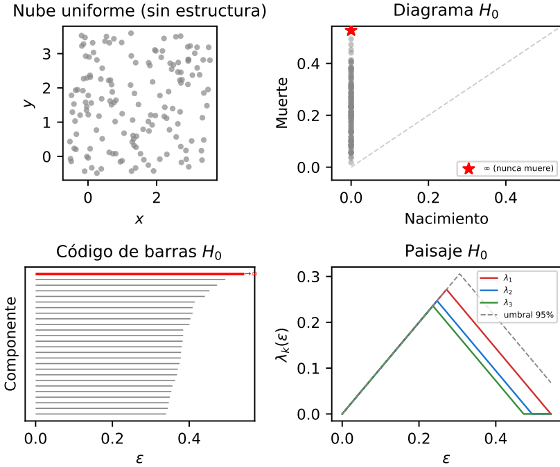
Figura 2.2: Control negativo: 150 puntos uniformes (sin estructura). El diagrama, el código de barras y el paisaje de persistencia muestran solo ruido — \lambda_1 apenas supera el umbral de hipótesis nula, sin los picos prominentes de la Figura 2.1.
