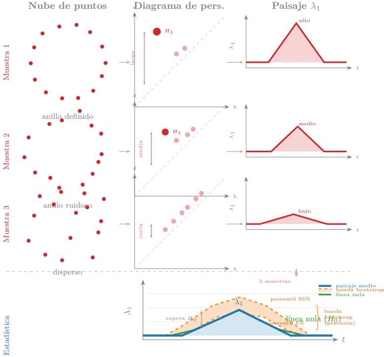
Figura 1.21: Tres muestras del mismo proceso (filas 1–3) producen diagramas de persistencia con barras de distinta longitud y paisajes con picos de distinta altura. La fila inferior superpone los tres paisajes individuales (rojo) para obtener el paisaje medio (azul), la banda bootstrap 5 %–95 % (naranja, banda de variabilidad de remuestras del dataset original) y la línea nula (verde, percentil 95 % de paisajes de datos permutados). El pico azul supera la línea nula — señal estadísticamente significativa — y queda dentro de la banda bootstrap — señal reproducible.
