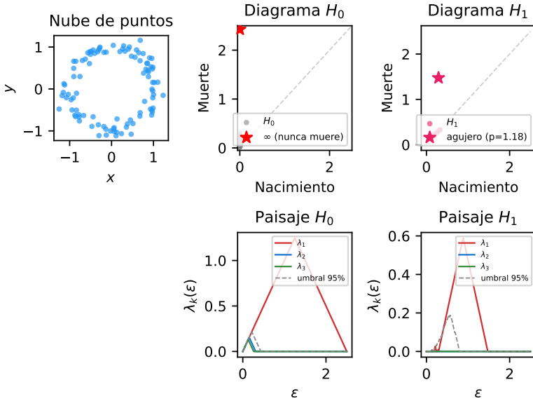
Figura 1.3: Receta 2: arriba, nube de puntos sobre un círculo con ruido, diagrama de persistencia H_0 y diagrama H_1 — la estrella rosa es el agujero central, lejos de la diagonal. Abajo, diagramas de paisajes con el umbral de hipótesis nula al 95 % de confianza (línea discontinua): en H_0 , \lambda_1 sobresale (la componente inmortal) pero \lambda_2 y \lambda_3 no — hay una sola pieza; en H_1 , \lambda_1 supera claramente el umbral, confirmando que el agujero es señal.
