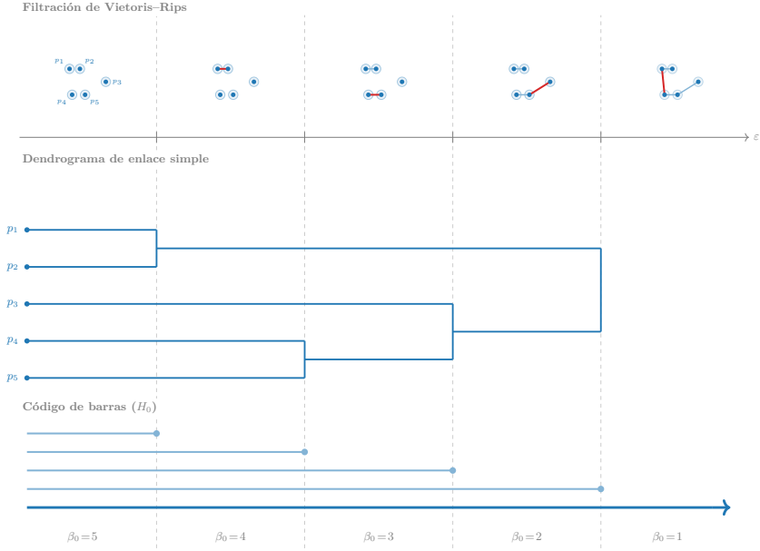
Figura 1.16: Filtración de Vietoris-Rips sobre cinco puntos (arriba), dendrograma de enlace simple (centro) y código de barras de H_0 (abajo), alineados por la misma escala \varepsilon . Cada fotograma muestra la arista que provoca la fusión (en rojo); el número \beta_0 indica cuántas componentes conexas quedan activas entre eventos. La barra inmortal (flecha) es la componente que persiste para siempre.
