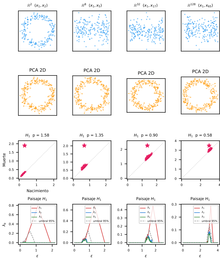
Figura 1.6: Maldición de la dimensionalidad: círculo de R = 1.5 embebido en \mathbb{R}^2 , \mathbb{R}^8 , \mathbb{R}^{32} y \mathbb{R}^{128} con ruido \sigma = 0.2 . Fila 1: proyección (x_1, x_{d/2+1}) — en alta dimensión, coordenada de ruido puro. Fila 2: PCA 2D — recupera el círculo siempre (escenario ideal para PCA). Fila 3: diagrama H_1 — la estrella más persistente se acerca a la diagonal. Fila 4: paisaje \lambda_1 — la razón señal/ruido decrece; en \mathbb{R}^{128} los picos de H_1 son difícilmente distinguibles del umbral de permutación.
