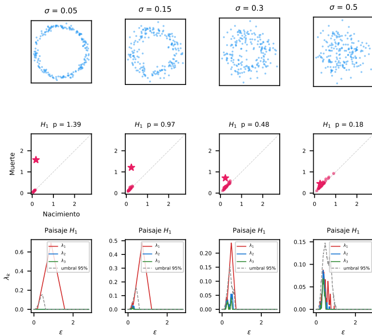
Figura 1.5: Receta 3 — estabilidad: arriba, el mismo círculo con cuatro niveles de ruido creciente ( \sigma ); centro, diagrama de persistencia H_1 (la estrella marca el agujero principal); abajo, paisaje de persistencia \lambda_1 con el umbral 95 %. La señal decrece gradualmente — nunca desaparece de golpe.
