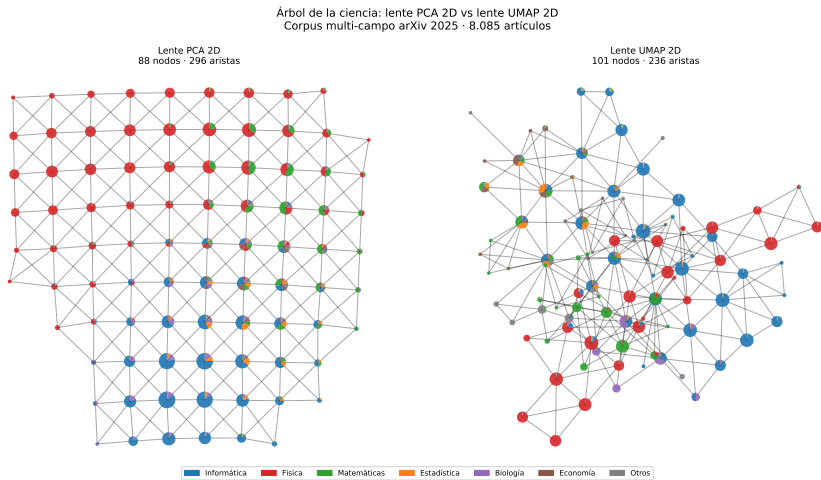
Figura 1.14: Receta 8 (árbol de la ciencia): comparación de lentes Mapper sobre el corpus arXiv 2025. Izquierda: lente PCA 2D con clustering PCA 20D — 88 nodos y 296 aristas. Derecha: lente UMAP 2D con DBSCAN coseno sobre \mathbb{R}^{384} — 101 nodos y 236 aristas. Con UMAP, las disciplinas se agrupan geográficamente según la variedad no lineal del corpus: los campos con vocabulario más similar aparecen contiguos, y los nodos multicolor (puentes interdisciplinarios) se concentran en las zonas de transición.
