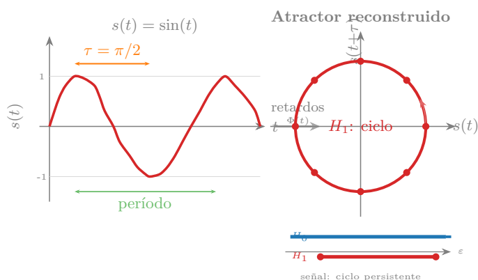
Figura 1.23: Embedding de retardos de s(t) = \sin(t) con retardo \tau = \pi/2 . Izquierda: la señal escalar s(t) vs. t . Derecha: la trayectoria (s(t), s(t+\tau)) en \mathbb{R}^2 traza un círculo limpio. El mini-barcode inferior muestra una componente inmortal en H_0 y un ciclo muy persistente en H_1 — la firma topológica de la periodicidad.
