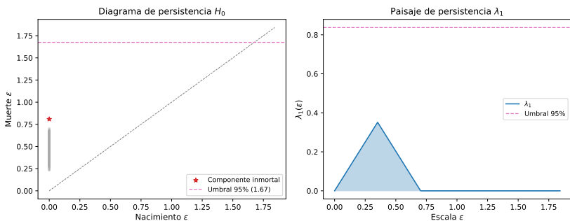
Figura 1.9: Análisis H_0 del corpus multi-campo (8.085 artículos de arXiv 2025, 29 categorías). Izquierda: diagrama de persistencia — todos los puntos cerca de la diagonal, ninguna barra supera el umbral del 95 %. Derecha: paisaje \lambda_1 con umbral nulo (línea discontinua). La ciencia arXiv es una única componente conexa a nivel de significación estadística.
