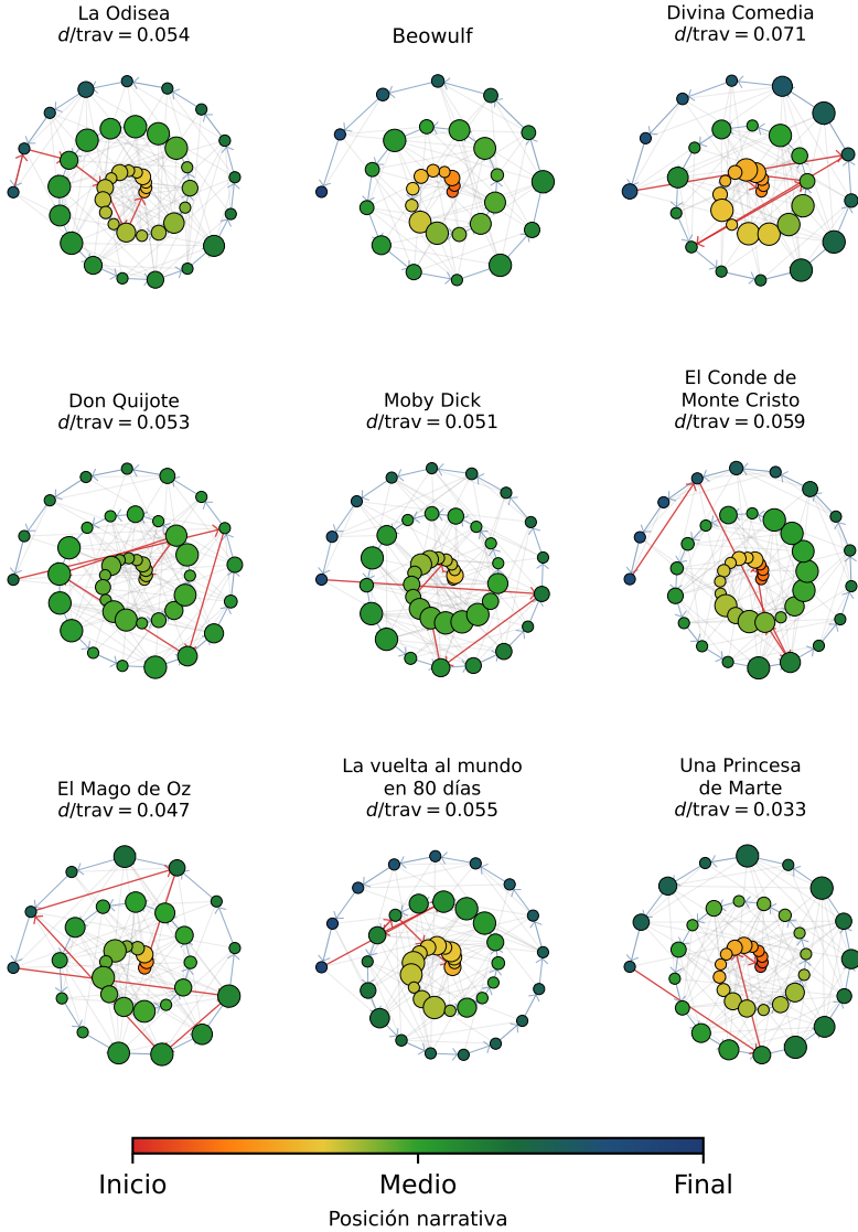
Figura 1.8: Receta 5: hipergrafo en espiral de nueve novelas clásicas. Cada nodo es un cluster semántico; su área es proporcional a la fracción de pasajes que contiene, y su posición en la espiral refleja el orden narrativo (centro = inicio, exterior = final). Flechas azules: recorrido cronológico. Flechas rojas: camino de retorno por aristas semánticas. El ratio d/trav mide el coste relativo del retorno.
