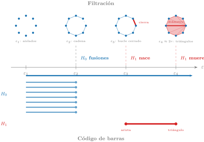
Figura 1.17: Cuatro fotografías de la filtración sincronizadas con el código de barras. \varepsilon_2 : las aristas forman una cadena ( \beta_0 = 1 , \beta_1 = 0 ). \varepsilon_3 : la arista roja cierra el bucle — H_1 nace ( \beta_1 = 1 ). \varepsilon_4 : cuando \varepsilon alcanza el diámetro ( 2r ), los triángulos en abanico —formados solo por puntos del anillo, sin punto central— rellenan el interior y H_1 muere ( \beta_1 = 0 ). El diámetro (línea roja gruesa) es la cuerda crítica.
