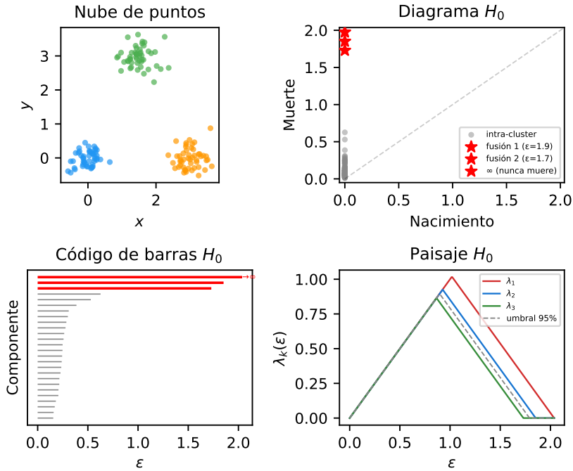
Figura 1.1: Receta 1: tres clusters gaussianos y tres representaciones equivalentes de su homología H_0 . Las tres estrellas rojas en el diagrama corresponden a los 3 clusters. En el paisaje de persistencia, los picos sobrepasan claramente el umbral de hipótesis nula (línea discontinua).
