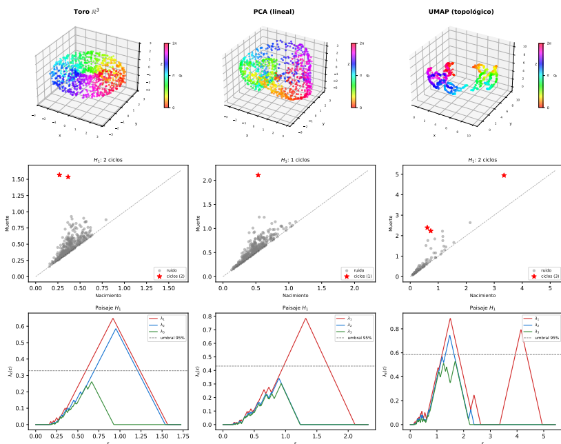
Figura 1.12: Receta 7: reducción de un toro ( \beta_1 = 2 ) desde \mathbb{R}^{50} a \mathbb{R}^3 con PCA (columna central) y UMAP (columna derecha), con el toro original en \mathbb{R}^3 como referencia (columna izquierda). Fila superior: nubes 3D coloreadas por \theta — PCA puede parecer geométricamente limpia, UMAP suele verse distorsionada: ambas apariencias son engañosas. Fila central: diagrama de persistencia H_1 , estrellas rojas = ciclos persistentes; PCA detecta 1, UMAP detecta 2. Fila inferior: paisaje de persistencia con capas \lambda_1 (rojo) y \lambda_2 (azul), umbral nulo al 95 % (línea discontinua) — solo UMAP tiene ambas capas sobre el umbral, confirmando \beta_1 = 2 .
