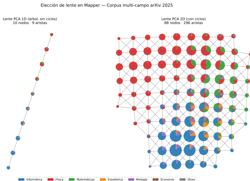
Figura 1.10: Comparación de lentes Mapper sobre el corpus arXiv 2025 (8.085 artículos). Izquierda: lente PCA 1D — árbol de 10 nodos y 9 aristas, sin ciclos. Derecha: lente PCA 2D — red de 88 nodos y 296 aristas con ciclos interdisciplinarios. La misma paleta de colores que en la Figura 1.11.
