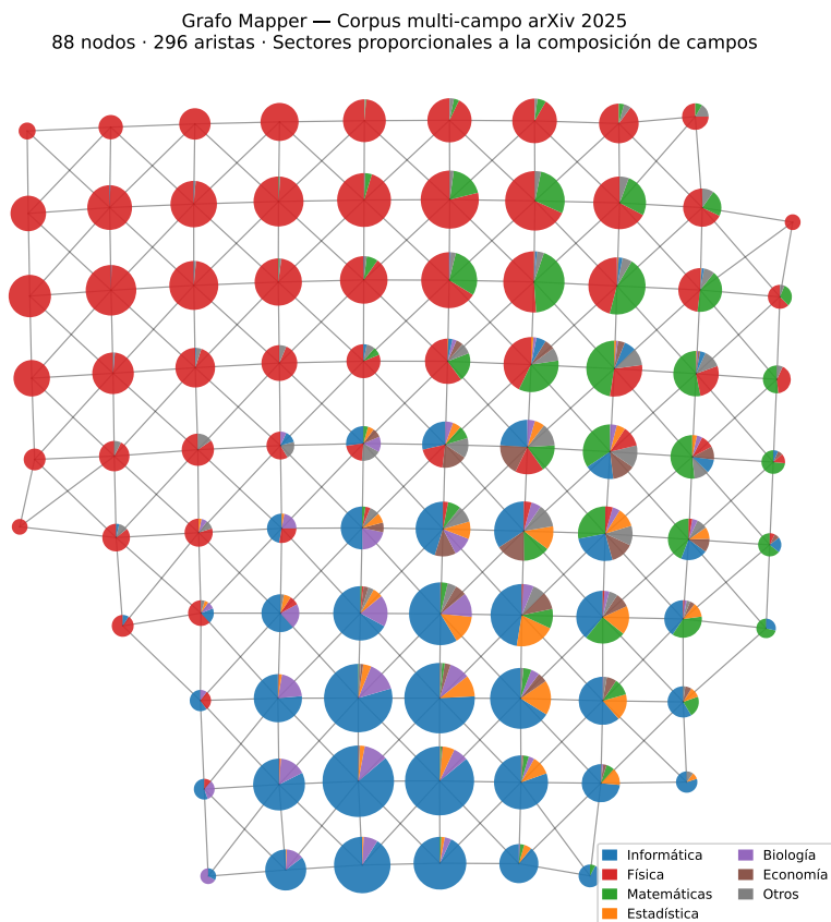
Figura 1.11: Grafo Mapper del corpus multi-campo arXiv 2025 (8.085 artículos, 88 nodos, lente PCA 2D). Cada nodo se dibuja como un pastel de sectores proporcionales a la composición de campos (azul = Informática, rojo = Física, verde = Matemáticas, naranja = Estadística, violeta = Biología, marrón = Economía). El tamaño es proporcional al número de papers. Los nodos de un único color son monodisciplinarios; los de varios colores son puentes interdisciplinarios.
