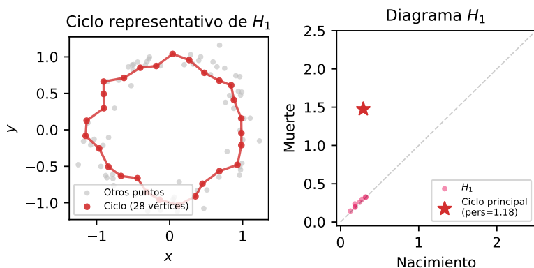
Figura 1.7: Receta 4: ciclo representativo del agujero principal. Izquierda: los vértices del ciclo (rojo) y sus aristas forman un polígono cerrado que encierra la región vacía central del anillo; los demás puntos aparecen en gris. Derecha: diagrama de persistencia H_1 con la estrella marcando la característica extraída.
