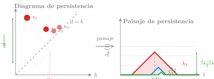
Figura 1.20: De diagrama de persistencia a paisaje. Cada punto (b_i, d_i) del PD genera una tienda de campaña \Lambda_i (panel izquierdo, coloreada por persistencia). El paisaje \lambda_k toma el k -ésimo máximo a cada escala t (panel derecho). Los niveles \lambda_1, \lambda_2, \lambda_3 capturan señal de persistencia decreciente: \lambda_1 refleja la característica dominante, \lambda_2 la secundaria.
