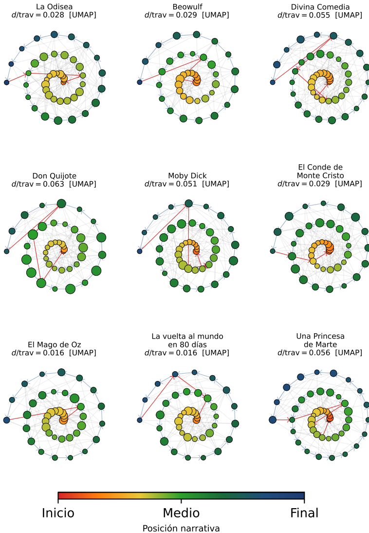
Figura 1.13: Receta 8 (camino del héroe): hipergrafo en espiral con lente UMAP 2D y DBSCAN con distancia coseno sobre los embeddings originales en \mathbb{R}^{384} . La lente no lineal organiza los parches del Mapper; los nodos se colocan en la espiral según su posición narrativa media (centro = inicio, exterior = final). Las flechas rojas (retorno) siguen cruzando casi todo el grafo, confirmando que el inicio y el final están semánticamente alejados en todas las novelas.
