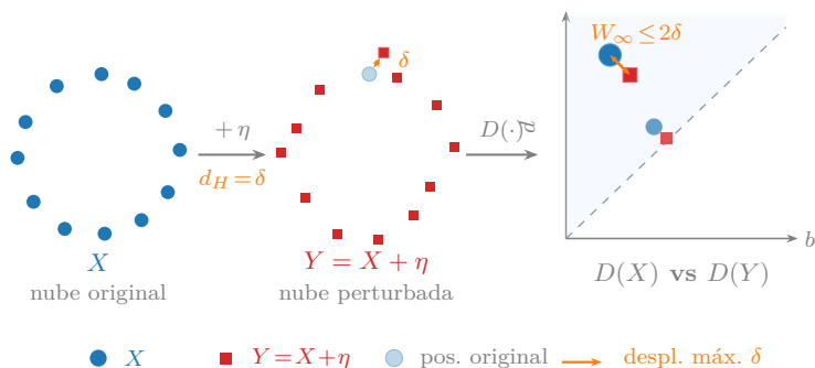
Figura 1.19: Ilustración del teorema de estabilidad en tres pasos. Izquierda: nube original X (puntos azules). Centro: nube perturbada Y = X + \eta ; el punto pálido muestra la posición original; la flecha naranja marca el peor desplazamiento \delta = d_H(X, Y) . Derecha: diagramas de persistencia D(X) (círculos) y D(Y) (cuadrados) superpuestos; las líneas grises muestran el emparejamiento bottleneck óptimo; la flecha naranja acota el mayor desplazamiento en el espacio de PDs, que no puede superar W_\infty \leq 2\delta .
