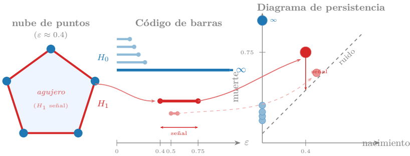
Figura 1.18: Izquierda: cinco puntos dispuestos en un pentágono regular a escala \varepsilon \approx 0.4 — las aristas (rojo) forman un bucle cerrado y el interior sombreado es el agujero que origina la característica H_1 . Centro: código de barras de la nube; las cuatro barras azules cortas son H_0 de ruido (componentes que se fusionan rápido), la barra azul larga con flecha es el H_0 inmortal, la barra roja larga es la señal H_1 (el agujero) y la barra roja muy corta es ruido H_1 . Derecha: diagrama de persistencia; los puntos azules pequeños cerca de la diagonal son ruido H_0 , el punto rojo grande alejado de la diagonal es la señal H_1 , y el punto rojo pequeño junto a la diagonal es el ruido H_1 . La distancia al eje diagonal mide la persistencia: señal arriba, ruido abajo. Las flechas muestran la correspondencia barra — punto.
