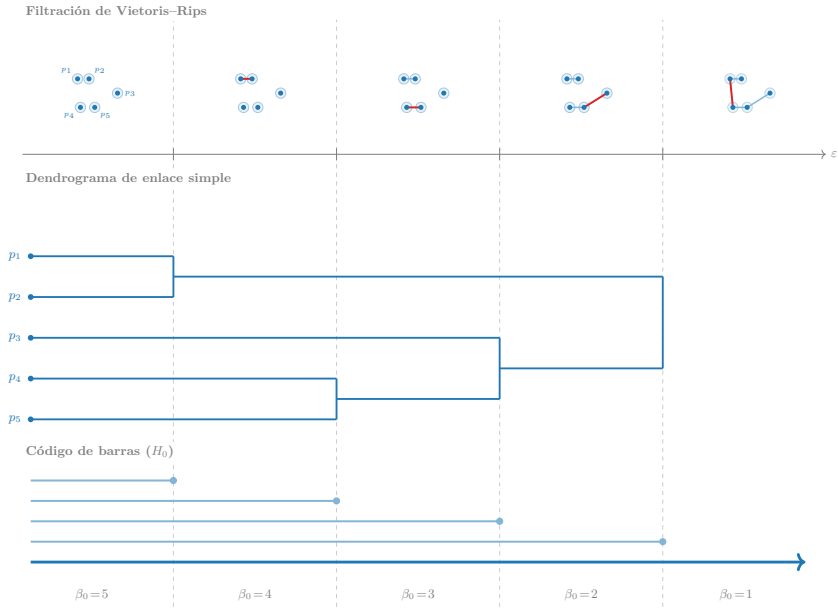
Figura 5.2: Filtración de Vietoris-Rips sobre cinco puntos (arriba), dendrograma de enlace simple (centro) y código de barras de H_0 (abajo), alineados por la misma escala \varepsilon . Cada fotograma muestra la arista que provoca la fusión (en rojo); el número \beta_0 indica cuántas componentes conexas quedan activas entre eventos. La barra inmortal (flecha) es la componente que persiste para siempre.
