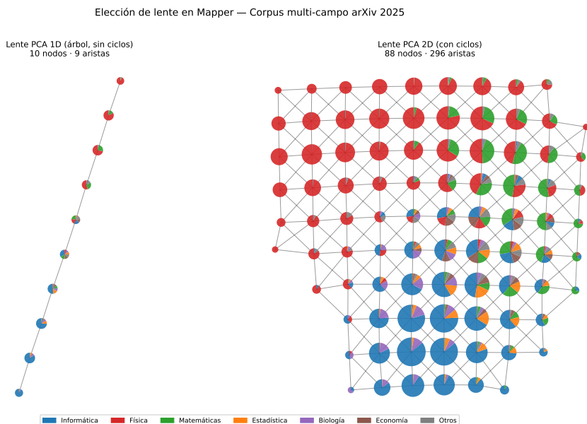
Figura 2.10: Comparación de lentes Mapper sobre el corpus arXiv 2025 (8.085 artículos). Izquierda: lente PCA 1D — árbol de 10 nodos y 9 aristas, sin ciclos. Derecha: lente PCA 2D — red de 88 nodos y 296 aristas con ciclos interdisciplinarios. La misma paleta de colores que en la Figura 2.11.
