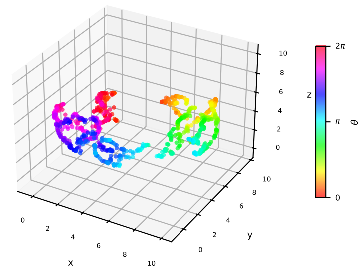
UMAP (topológico)
