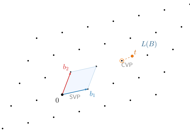
Figura 3.1: Retículo bidimensional generado por dos vectores base b_1 y b_2 . La región sombreada es el dominio fundamental (paralelogramo definido por la base). El punto t está fuera del retículo: encontrar el punto del retículo más cercano (CVP) o el vector no nulo más corto (SVP) es computacionalmente intratable en dimensiones altas.
