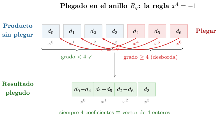
Figura 3.2: Plegado en el anillo R_q . Al multiplicar polinomios, los términos de grado mayor o igual que n se pliegan al rango [0, n-1] mediante la regla x^n = -1 . Esta restricción equivale a trabajar con matrices anticirculantes, codificando una matriz de n \times n enteros en solo n coeficientes.
