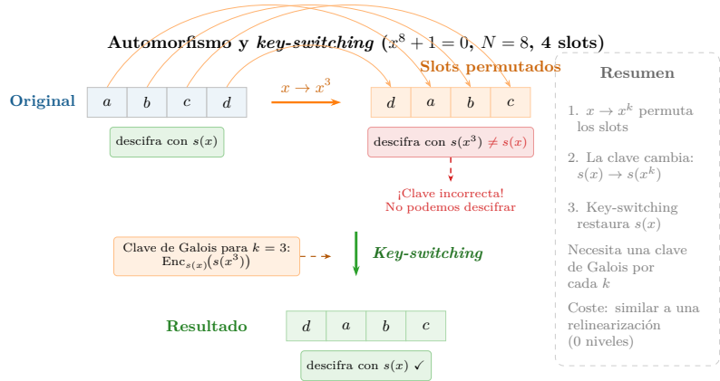
Figura 3.13: Automorfismo y key-switching (ejemplo con x^8 + 1 = 0 , N = 8 , 4 slots). La sustitución x \rightarrow x^3 permuta cíclicamente los slots: [a, b, c, d] \rightarrow [d, a, b, c] . Pero cambia la clave de descifrado de s(x) a s(x^3) . El key-switching, usando una clave de Galois precalculada, restaura la clave original sin revelar el secreto.
