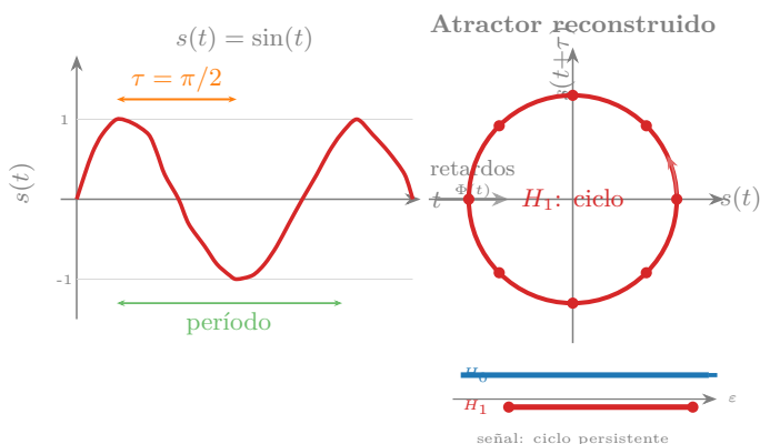
Figura 22.24: Embedding de retardos de s(t) = \sin(t) con retardo \tau = \pi/2 . Izquierda: la señal escalar s(t) vs. t . Derecha: la trayectoria (s(t), s(t+\tau)) en \mathbb{R}^2 traza un círculo limpio. El mini-barcode inferior muestra una componente inmortal en H_0 y un ciclo muy persistente en H_1 — la firma topológica de la periodicidad.
