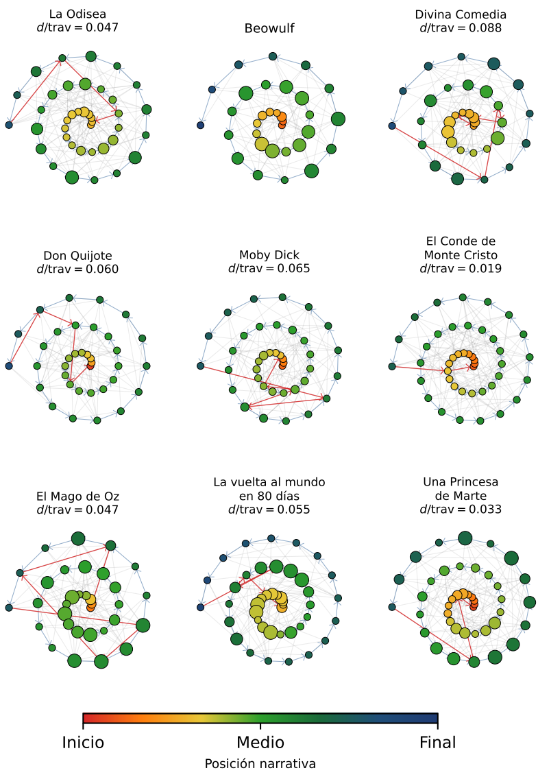
Figura 22.8: Receta 5: hipergrafo en espiral de nueve novelas clásicas. Cada nodo es un cluster semántico; su área es proporcional a la fracción de pasajes que contiene, y su posición en la espiral refleja el orden narrativo (centro = inicio, exterior = final). Flechas azules: recorrido cronológico. Flechas rojas: camino de retorno por aristas semánticas. El ratio d/trav mide el coste relativo del retorno.
