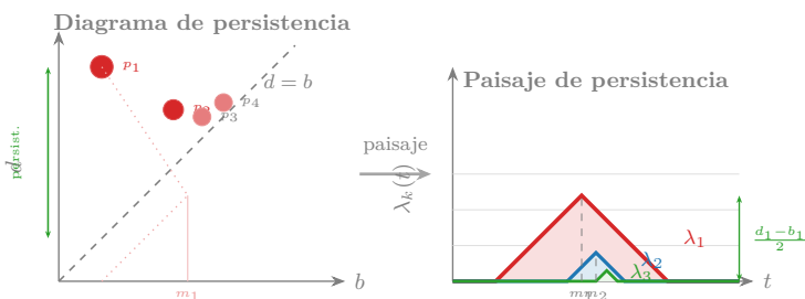
Figura 22.21: De diagrama de persistencia a paisaje. Cada punto (b_i, d_i) del PD genera una tienda de campaña \Lambda_i (panel izquierdo, coloreada por persistencia). El paisaje \lambda_k toma el k -ésimo máximo a cada escala t (panel derecho). Los niveles \lambda_1, \lambda_2, \lambda_3 capturan señal de persistencia decreciente: \lambda_1 refleja la característica dominante, \lambda_2 la secundaria.
