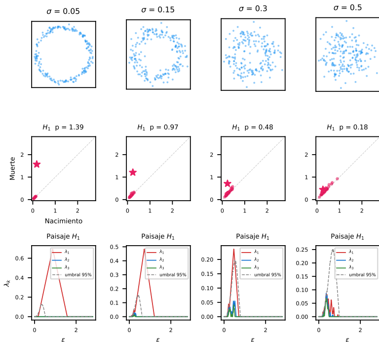
Figura 22.5: Receta 3 — estabilidad: arriba, el mismo círculo con cuatro niveles de ruido creciente ( \sigma ); centro, diagrama de persistencia H_1 (la estrella marca el agujero principal); abajo, paisaje de persistencia \lambda_1 con el umbral 95 %. La señal decrece gradualmente — nunca desaparece de golpe.
