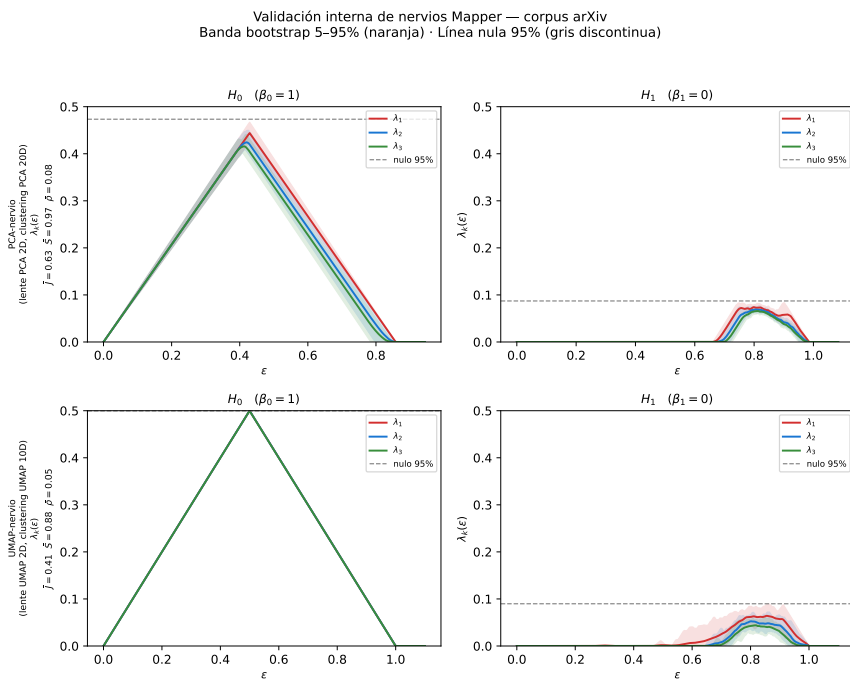
Figura 22.15: Validación interna de los dos nervios Mapper sobre el corpus arXiv. Cada panel muestra el paisaje de persistencia medio (líneas) con la banda bootstrap 5–95 % (sombreado) y la línea nula al 95 % (gris discontinua) para H_0 y H_1 . H_2 no se calcula: con lente 2D es estructuralmente nula (ver Sección 22.6.8). La leyenda de cada fila incluye \bar{J} , \bar{S} y \rho (densidad media del nervio bootstrap, parámetro del modelo binomial nulo utilizado para calcular el z-score de \bar{S} ).
