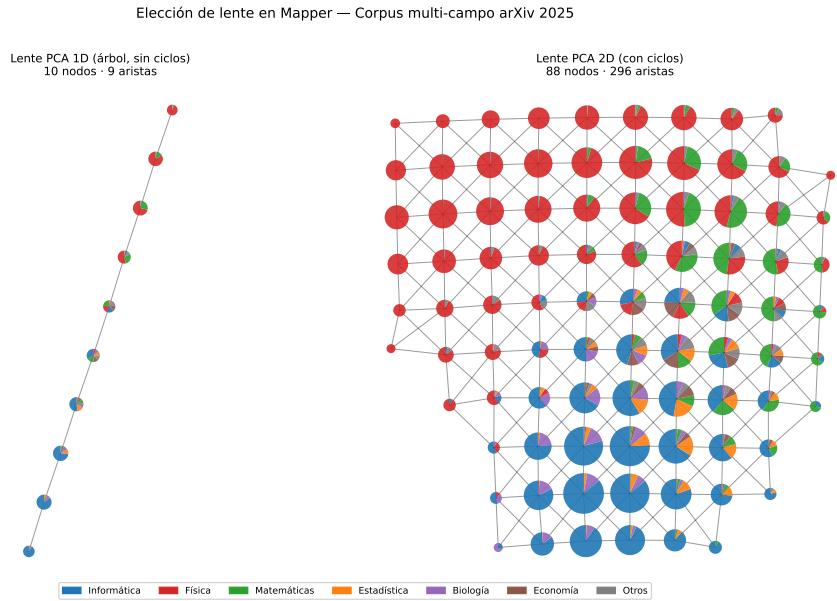
Figura 22.10: Comparación de lentes Mapper sobre el corpus arXiv 2025 (8.085 artículos). Izquierda: lente PCA 1D — árbol de 10 nodos y 9 aristas, sin ciclos. Derecha: lente PCA 2D — red de 88 nodos y 296 aristas con ciclos interdisciplinarios. La misma paleta de colores que en la Figura 22.11.
