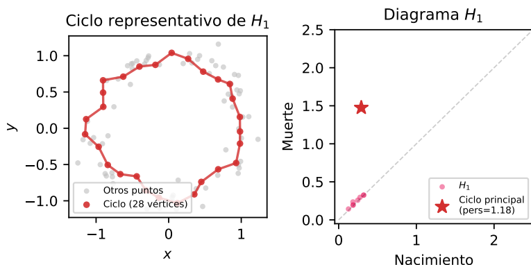
Figura 22.7: Receta 4: ciclo representativo del agujero principal. Izquierda: los v rtices del ciclo (rojo) y sus aristas forman un pol gono cerrado que encierra la regi n vac a central del anillo; los dem s puntos aparecen en gris. Derecha: diagrama de persistencia H_1 con la estrella marcando la caracter stica extra da.
