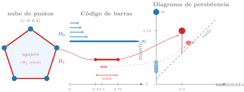
Figura 22.19: Izquierda: cinco puntos dispuestos en un pentágono regular a escala \varepsilon \approx 0.4 — las aristas (rojo) forman un bucle cerrado y el interior sombreado es el agujero que origina la característica H_1 . Centro: código de barras de la nube; las cuatro barras azules cortas son H_0 de ruido (componentes que se fusionan rápido), la barra azul larga con flecha es el H_0 inmortal, la barra roja larga es la señal H_1 (el agujero) y la barra roja muy corta es ruido H_1 . Derecha: diagrama de persistencia; los puntos azules pequeños cerca de la diagonal son ruido H_0 , el punto rojo grande alejado de la diagonal es la señal H_1 , y el punto rojo pequeño junto a la diagonal es el ruido H_1 . La distancia al eje diagonal mide la persistencia: señal arriba, ruido abajo. Las flechas muestran la correspondencia barra — punto.
