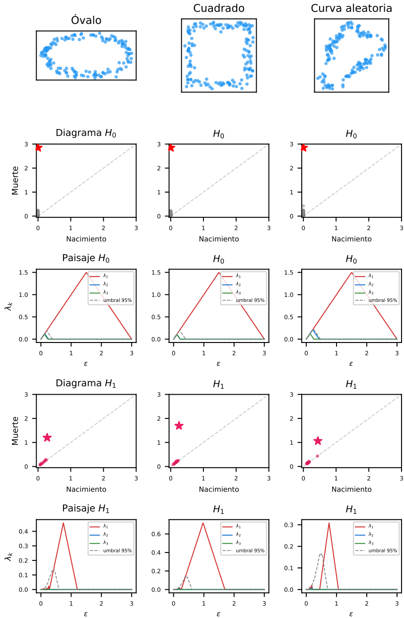
Figura 22.4: Invarianza topológica: un óvalo, un cuadrado y una curva aleatoria — tres geometrías distintas con la misma topología. En todos los casos, H_0 detecta una componente y H_1 detecta un ciclo persistente (estrella). La forma geométrica cambia; la forma topológica, no.
