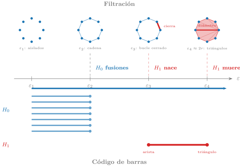
Figura 22.18: Cuatro fotografías de la filtración sincronizadas con el código de barras. \varepsilon_2 : las aristas forman una cadena ( \beta_0 = 1 , \beta_1 = 0 ). \varepsilon_3 : la arista roja cierra el bucle — H_1 nace ( \beta_1 = 1 ). \varepsilon_4 : cuando \varepsilon alcanza el diámetro ( 2r ), los triángulos en abanico —formados solo por puntos del anillo, sin punto central— rellenan el interior y H_1 muere ( \beta_1 = 0 ). El diámetro (línea roja gruesa) es la cuerda crítica.
