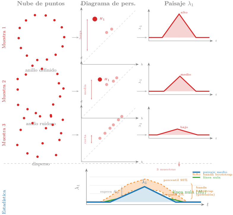
Figura 22.22: Tres muestras del mismo proceso (filas 1–3) producen diagramas de persistencia con barras de distinta longitud y paisajes con picos de distinta altura. La fila inferior superpone los tres paisajes individuales (rojo) para obtener el paisaje medio (azul), la banda bootstrap 5 %–95 % (naranja, banda de variabilidad de remuestras del dataset original) y la línea nula (verde, percentil 95 % de paisajes de datos permutados). El pico azul supera la línea nula — señal estadísticamente significativa — y queda dentro de la banda bootstrap — señal reproducible.
