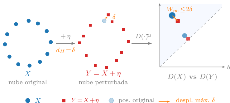
Figura 22.20: Ilustración del teorema de estabilidad en tres pasos. Izquierda: nube original X (puntos azules). Centro: nube perturbada Y = X + \eta ; el punto pálido muestra la posición original; la flecha naranja marca el peor desplazamiento \delta = d_H(X, Y) . Derecha: diagramas de persistencia D(X) (círculos) y D(Y) (cuadrados) superpuestos; las líneas grises muestran el emparejamiento bottleneck óptimo; la flecha naranja acota el mayor desplazamiento en el espacio de PDs, que no puede superar W_\infty \leq 2\delta .
