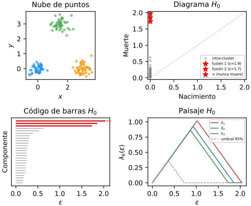
Figura 22.1: Receta 1: tres clusters gaussianos y tres representaciones equivalentes de su homología H_0 . Las tres estrellas rojas en el diagrama corresponden a los 3 clusters. En el paisaje de persistencia, los picos sobrepasan claramente el umbral nulo (línea discontinua).
