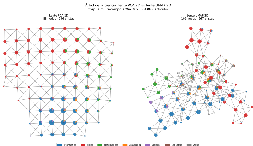
Figura 22.14: Receta 8 (árbol de la ciencia): comparación de lentes Mapper sobre el corpus arXiv 2025. Izquierda: lente PCA 2D con clustering PCA 20D — 88 nodos y 296 aristas. Derecha: lente UMAP 2D con clustering UMAP 10D — 106 nodos y 267 aristas. Con UMAP, las disciplinas se agrupan geográficamente según la variedad no lineal del corpus: los campos con vocabulario más similar aparecen contiguos, y los nodos multicolor (puentes interdisciplinarios) se concentran en las zonas de transición.
