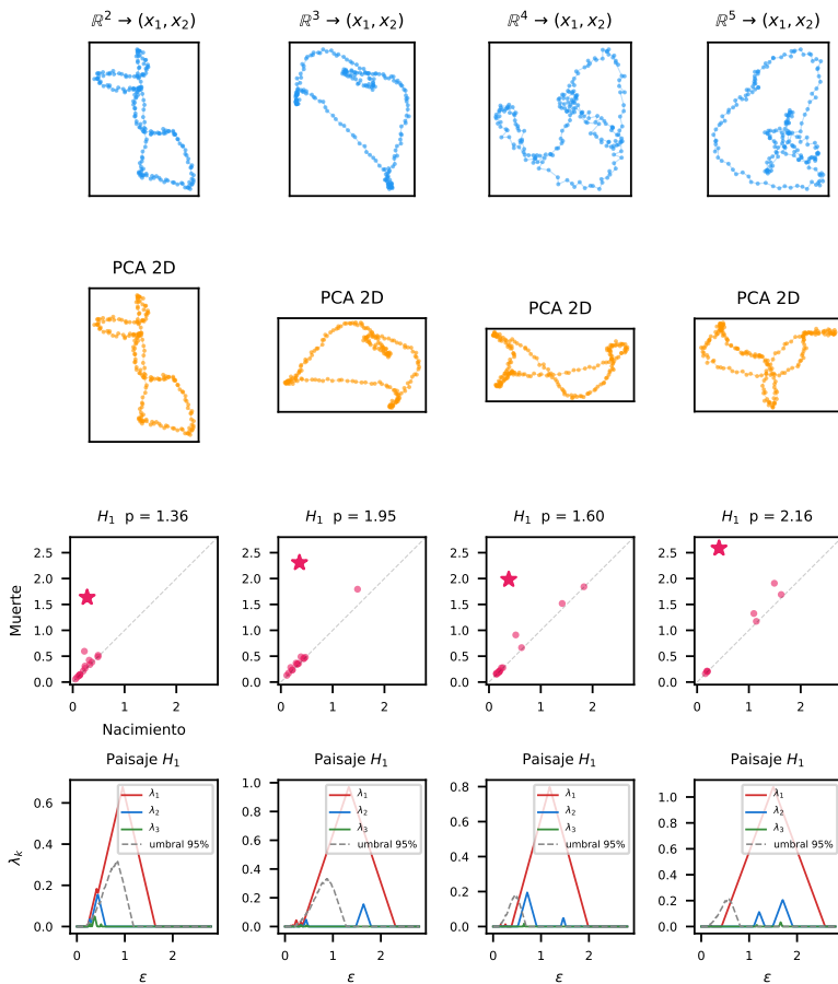
Figura 22.6: Invarianza topológica: bucles cerrados aleatorios (series de Fourier, 200 puntos) en \mathbb{R}^2 , \mathbb{R}^3 , \mathbb{R}^4 y \mathbb{R}^5 . Fila 1: proyección en (x_1, x_2) — formas distorsionadas. Fila 2: PCA 2D — revela el bucle. Fila 3: diagramas H_1 — un ciclo persistente en todos los casos (estrella). Fila 4: paisajes \lambda_1 — superan el umbral 95 %.
