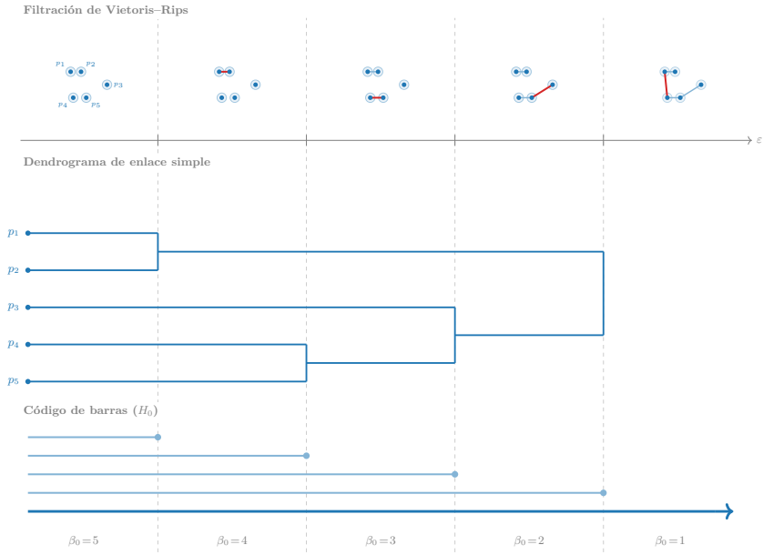
Figura 22.17: Filtración de Vietoris-Rips sobre cinco puntos (arriba), dendrograma de enlace simple (centro) y código de barras de H_0 (abajo), alineados por la misma escala \varepsilon . Cada fotograma muestra la arista que provoca la fusión (en rojo); el número \beta_0 indica cuántas componentes conexas quedan activas entre eventos. La barra inmortal (flecha) es la componente que persiste para siempre.
