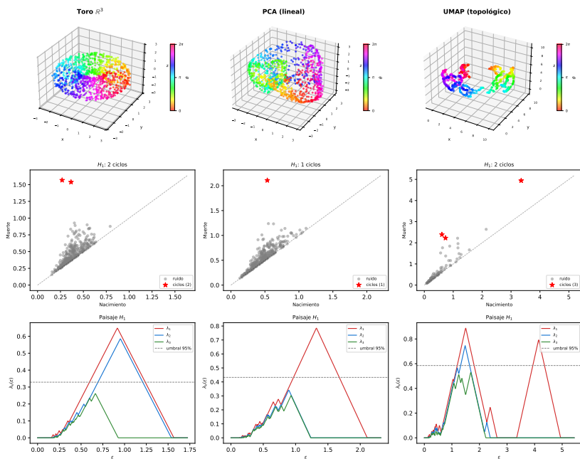
Figura 22.12: Receta 7: reducción de un toro ( \beta_1 = 2 ) desde \mathbb{R}^{50} a \mathbb{R}^3 con PCA (columna central) y UMAP (columna derecha), con el toro original en \mathbb{R}^3 como referencia (columna izquierda). Fila superior: nubes 3D coloreadas por \theta — PCA puede parecer geométricamente limpia, UMAP suele verse distorsionada: ambas apariencias son engañosas. Fila central: diagrama de persistencia H_1 , estrellas rojas = ciclos persistentes; PCA detecta 1, UMAP detecta 2. Fila inferior: paisaje de persistencia con capas \lambda_1 (rojo) y \lambda_2 (azul), umbral nulo al 95 % (línea discontinua) — solo UMAP tiene ambas capas sobre el umbral, confirmando \beta_1 = 2 .
