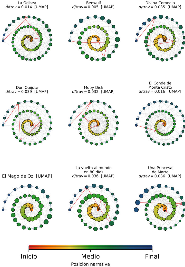
Figura 22.13: Receta 8 (camino del héroe): hipergrafo en espiral con lente UMAP 2D y clustering UMAP 10D, ambas reducciones independientes. La lente no lineal agrupa en cada parche pasajes que PCA separaría; los nodos se colocan en la espiral según su posición narrativa media (centro = inicio, exterior = final). Las flechas rojas (retorno) siguen cruzando casi todo el grafo, confirmando que el inicio y el final están semánticamente alejados en todas las novelas.
