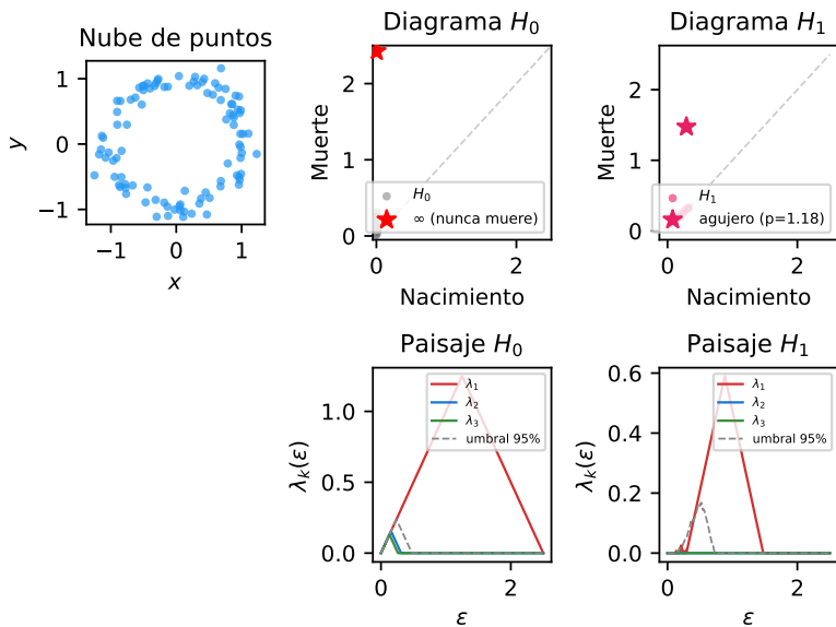
Figura 22.3: Receta 2: arriba, nube de puntos sobre un círculo con ruido, diagrama de persistencia H_0 y diagrama H_1 — la estrella rosa es el agujero central, lejos de la diagonal. Abajo, landscapes con el umbral 95 % (línea discontinua): en H_0 , \lambda_1 sobresale (la componente inmortal) pero \lambda_2 y \lambda_3 no — hay una sola pieza; en H_1 , \lambda_1 supera claramente el umbral, confirmando que el agujero es señal.
