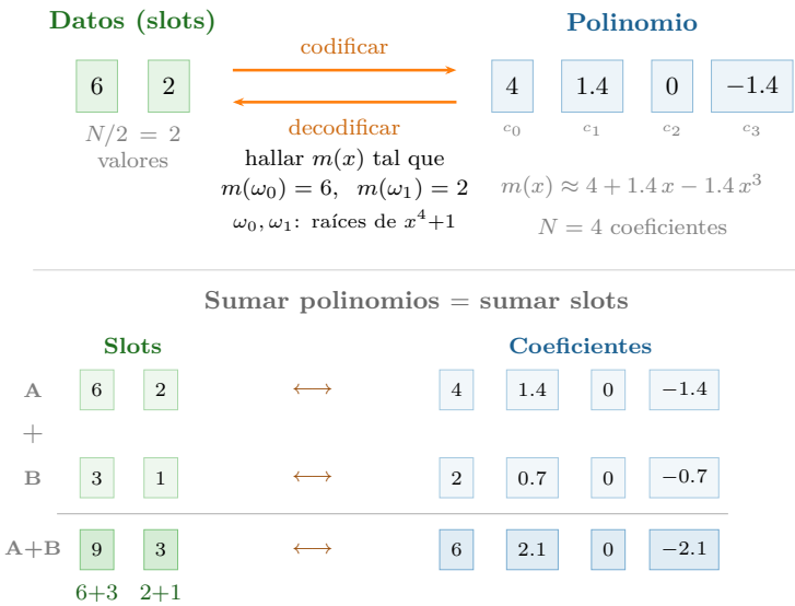
Figura 4.11: Codificación por slots ( N = 4 ). Arriba: dos datos [6, 2] se codifican como un polinomio de 4 coeficientes hallando m(x) tal que m(\omega_0) = 6 y m(\omega_1) = 2 . Abajo: sumar dos polinomios coeficiente a coeficiente equivale a sumar los slots dato a dato — la base del paralelismo SIMD.
