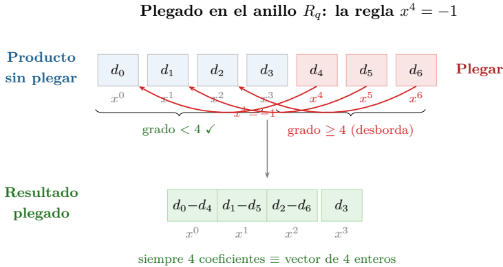
Figura 4.2: Plegado en el anillo R_q . Al multiplicar polinomios, los términos de grado mayor o igual que n se pliegan al rango [0, n - 1] mediante la regla x^n = -1 . Esta restricción equivale a trabajar con matrices anticirculantes, codificando una matriz de n \times n enteros en solo n coeficientes.
