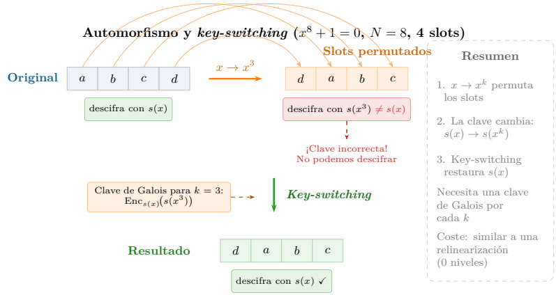
Figura 4.13: Automorfismo y key-switching (ejemplo con x^8 + 1 = 0 , N = 8 , 4 slots). La sustitución x \rightarrow x^3 permuta cíclicamente los slots: [a, b, c, d] \rightarrow [d, a, b, c] . Pero cambia la clave de descifrado de s(x) a s(x^3) . El key-switching, usando una clave de Galois precalculada, restaura la clave original sin revelar el secreto.
