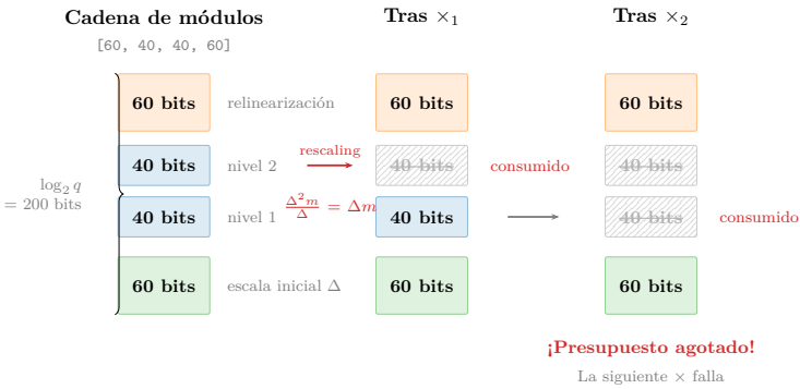
Figura 4.7: Cadena de módulos y consumo de niveles. Cada multiplicación consume un eslabón de 40 bits mediante rescaling. Cuando se agotan los eslabones intermedios, la siguiente multiplicación falla.
