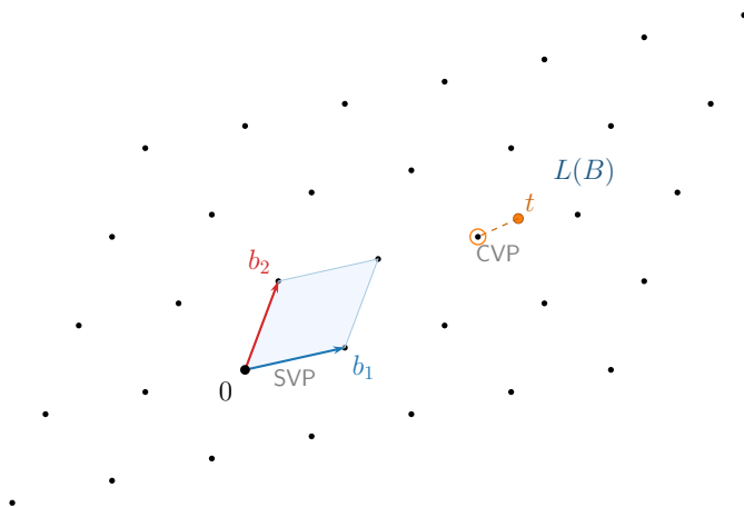
Figura 4.1: Retículo bidimensional generado por dos vectores base b_1 y b_2 . La región sombreada es el dominio fundamental (paralelogramo definido por la base). El punto t está fuera del retículo: encontrar el punto del retículo más cercano (CVP) o el vector no nulo más corto (SVP) es computacionalmente intratable en dimensiones altas.
