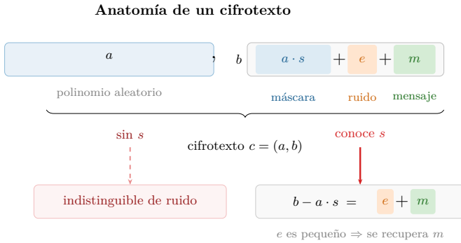
Figura 4.4: Anatomía de un cifrotexto. El par (a, b) contiene el mensaje m oculto tras una máscara a \cdot s y un ruido e . Quien conoce s elimina la máscara y recupera m ; sin s , el cifrotexto es indistinguible de ruido aleatorio.
