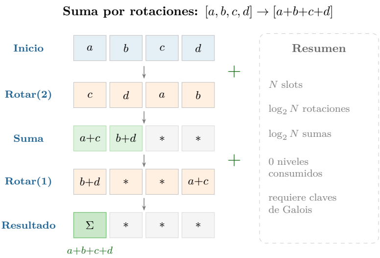
Figura 4.12: Suma por rotaciones. Con 4 slots, dos pasos de rotar-y-sumar bastan para acumular la suma total en el primer slot. El diagrama muestra la vista por slots; internamente, cada «Suma» es una adición de los N coeficientes de dos polinomios, que por linealidad de la evaluación produce la suma slot a slot. Las rotaciones requieren claves de Galois, pero no consumen niveles multiplicativos.
