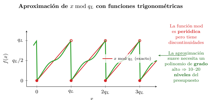
Figura 4.8: Aproximación de la reducción modular. La función « x módulo q_L » es periódica pero discontinua — no se puede expresar como una secuencia de sumas y multiplicaciones. Para evaluarla homomórficamente se aproxima mediante un polinomio de grado alto, que consume entre 10 y 20 niveles multiplicativos.
