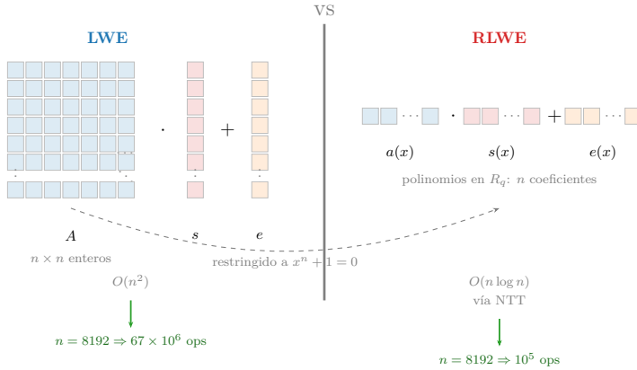
Figura 4.3: LWE frente a RLWE. A la izquierda, LWE requiere una matriz A de n \times n enteros. A la derecha, RLWE codifica la misma información en un polinomio de n coeficientes, reduciendo el coste de O(n^2) a O(n \log n) vía la NTT.
