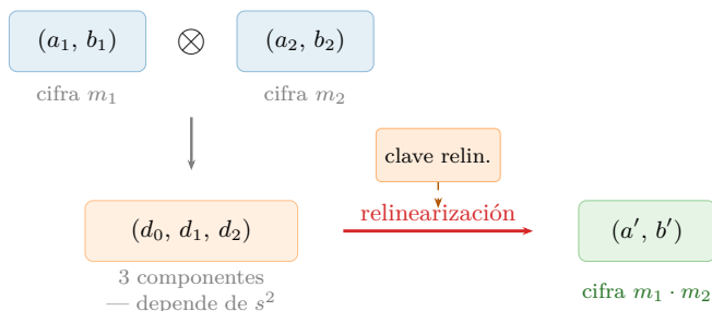
Figura 4.5: Multiplicación entre cifrotextos. El producto genera un triplete (d_0, d_1, d_2) que depende de s^2 . La relinearización, usando una clave pública que cifra s^2 , lo reduce a un par estándar (a', b') descifrable con s .
