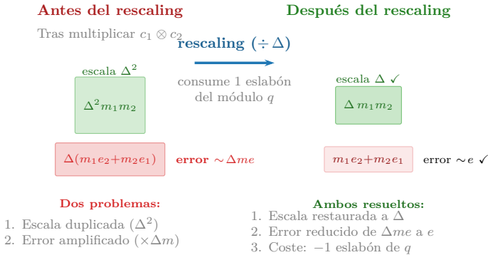
Figura 4.6: Rescaling: dividir por \Delta corrige simultáneamente la escala duplicada y el error amplificado, a cambio de consumir un eslabón de la cadena de módulos.
