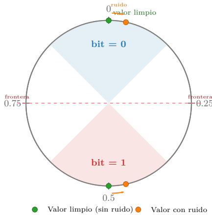
Figura 4.14: Codificación en el toro \mathbb{T} = \mathbb{R}/\mathbb{Z} . El bit 0 se codifica cerca de 0.0 (arriba) y el bit 1 cerca de 0.5 (abajo). El ruido desplaza la posición, pero el bit se recupera mientras no cruce la frontera de decisión.
