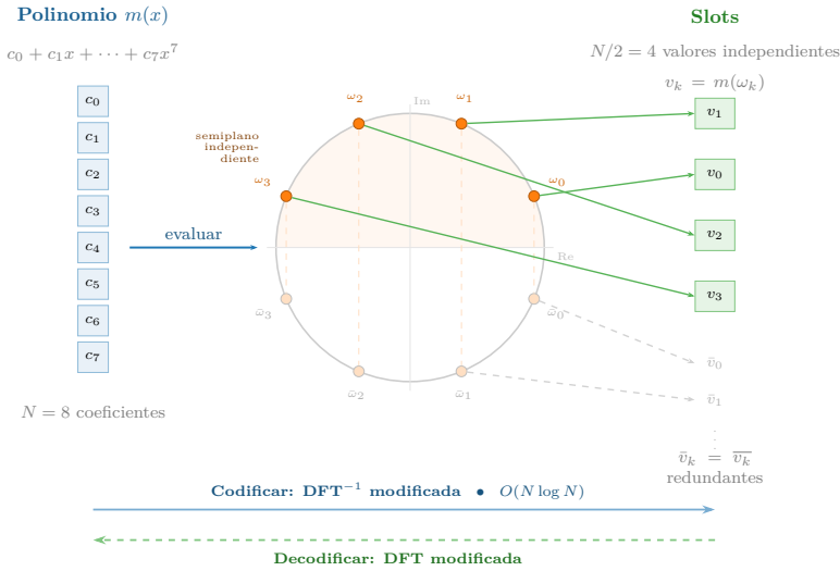
Figura 4.10: Inmersión canónica. Los coeficientes del polinomio m(x) no son los datos: los slots son las evaluaciones de m(x) en las N raíces complejas de x^N + 1 . Las raíces conjugadas producen valores redundantes, dejando N/2 slots independientes. Codificar y decodificar equivale a una DFT modificada (inversa y directa, respectivamente).
