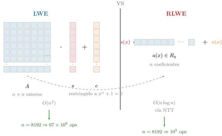
Figura 3.3: LWE frente a RLWE. A la izquierda, LWE requiere una matriz A de n \times n enteros. A la derecha, RLWE codifica la misma información en un polinomio de n coeficientes, reduciendo el coste de O(n^2) a O(n \log n) vía la NTT.
