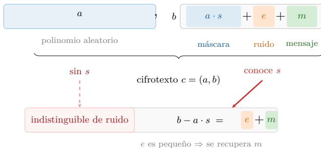
Figura 3.4: Anatomía de un cifrotexto. El par (a, b) contiene el mensaje m oculto tras una máscara a \cdot s y un ruido e . Quien conoce s elimina la máscara y recupera m ; sin s , el cifrotexto es indistinguible de ruido aleatorio.
