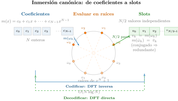
Figura 3.10: Inmersión canónica. Los coeficientes del polinomio m(x) no son los datos: los slots son las evaluaciones de m(x) en las N raíces complejas de x^N + 1 . Las raíces conjugadas producen valores redundantes, dejando N/2 slots independientes. Codificar y decodificar equivale a una DFT inversa y directa, respectivamente.
