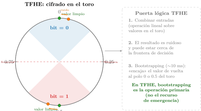
Figura 3.14: TFHE: cifrado en el toro. El valor descifrado cae en un punto de un círculo de 0 a 1. El bit 0 se codifica cerca del polo superior (0) y el bit 1 cerca del inferior (0.5). El ruido desplaza el valor, pero mientras no cruce la frontera de decisión, el bit se recupera. El bootstrapping restaura la posición en cada puerta lógica.
