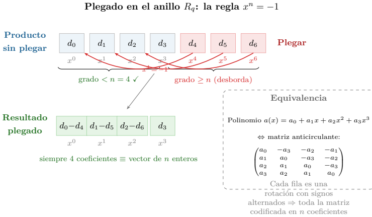
Figura 3.2: Plegado en el anillo R_q . Al multiplicar polinomios, los términos de grado mayor o igual que n se plegan al rango [0, n-1] mediante la regla x^n = -1 . Esta restricción equivale a trabajar con matrices anticirculantes, codificando una matriz de n \times n enteros en solo n coeficientes.
