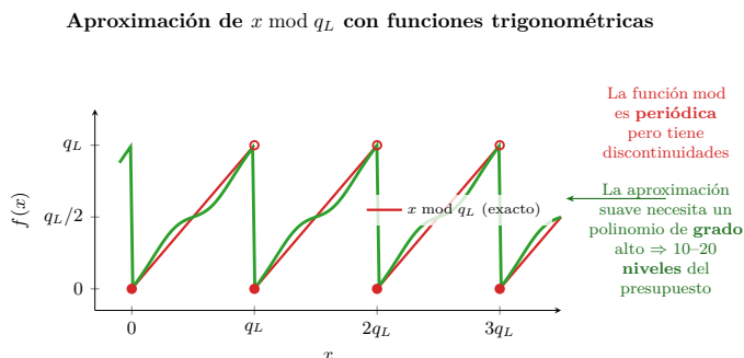
Figura 3.8: Aproximación de la reducción modular. La función « x módulo q_L » es periódica pero discontinua, y no se puede expresar como un polinomio. Para evaluarla homomórficamente se aproxima con funciones trigonométricas suaves, lo que requiere un polinomio de grado alto que consume entre 10 y 20 niveles multiplicativos.
