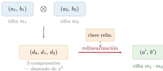
Figura 3.5: Multiplicación entre cifrotextos. El producto genera un triplete (d_0, d_1, d_2) que depende de s^2 . La relinearización, usando una clave pública que cifra s^2 , lo reduce a un par estándar (a', b') descifrable con s .
