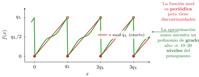
Figura 3.8: Aproximación de la reducción modular. La función « x módulo q_L » es periódica pero discontinua — no se puede expresar como una secuencia de sumas y multiplicaciones. Para evaluarla homomórficamente se aproxima mediante un polinomio de grado alto, que consume entre 10 y 20 niveles multiplicativos.
