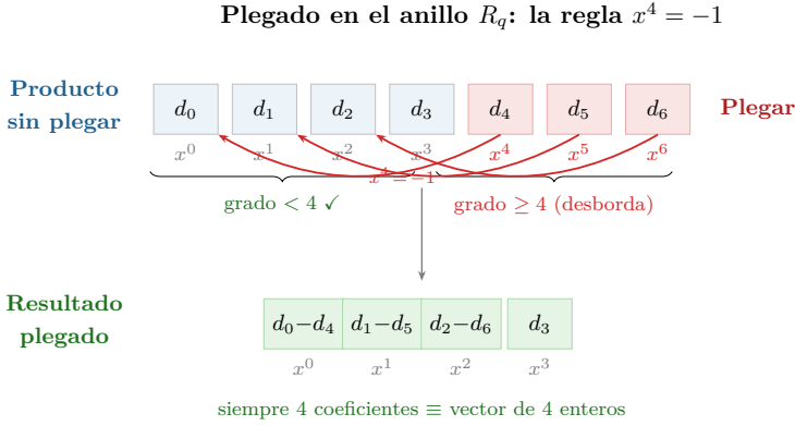
Figura 3.2: Plegado en el anillo R_q . Al multiplicar polinomios, los términos de grado mayor o igual que n se pliegan al rango [0, n - 1] mediante la regla x^n = -1 . Esta restricción equivale a trabajar con matrices anticirculantes, codificando una matriz de n \times n enteros en solo n coeficientes.
