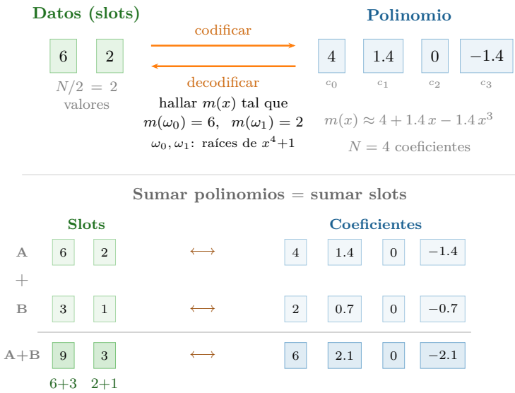
Figura 3.11: Codificación por slots ( N = 4 ). Arriba: dos datos [6, 2] se codifican como un polinomio de 4 coeficientes hallando m(x) tal que m(\omega_0) = 6 y m(\omega_1) = 2 . Abajo: sumar dos polinomios coeficiente a coeficiente equivale a sumar los slots dato a dato — la base del paralelismo SIMD.
