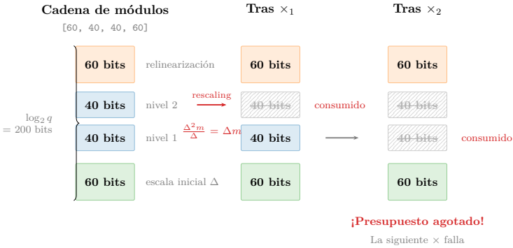
Figura 3.7: Cadena de módulos y consumo de niveles. Cada multiplicación consume un eslabón de 40 bits mediante rescaling. Cuando se agotan los eslabones intermedios, la siguiente multiplicación falla.
