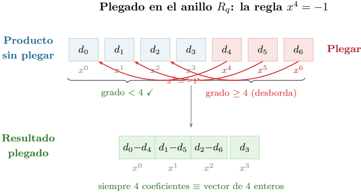
Figura 3.2: Plegado en el anillo R_q . Al multiplicar polinomios, los términos de grado mayor o igual que n se pliegan al rango [0, n-1] mediante la regla x^n = -1 . Esta restricción equivale a trabajar con matrices anticirculantes, codificando una matriz de n \times n enteros en solo n coeficientes.
