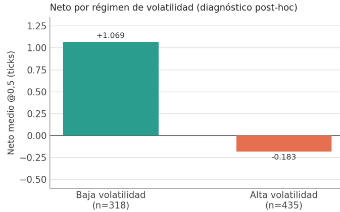
Figura 4.2: Contraste post-hoc del neto medio entre baja y alta volatilidad. La separación es una hipótesis de política que requiere datos posteriores.
