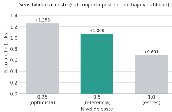
Figura 4.3: Sensibilidad al coste del subconjunto de baja volatilidad. Resultado exploratorio obtenido tras inspeccionar el mismo bloque.
