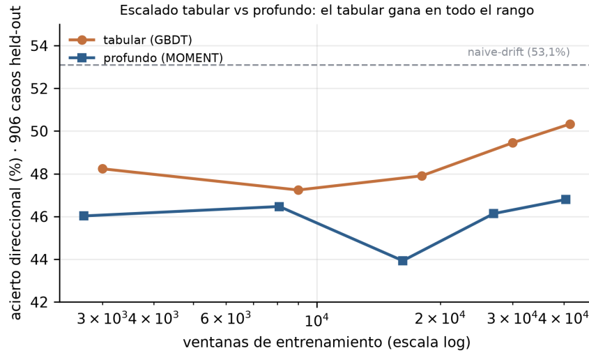
Figura 4.9: Curva de escalado sobre la misma tarea (dirección H60, 906 casos congelados): la vía tabular ( gradient boosting ) supera a la profunda (MOMENT) en todo el presupuesto de datos, y la distancia se mantiene o crece al aumentar el número de ventanas de entrenamiento. Con este horizonte de datos, más muestras no hacen que el aprendizaje profundo alcance al tabular.
