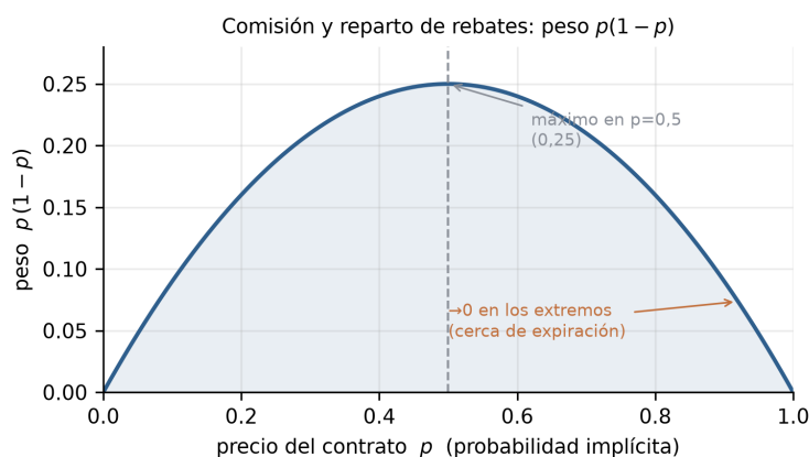
Figura 5.1: El peso p(1-p) que gobierna la comisión taker y el reparto de rebates al maker: máximo en p = 0,5 y nulo en los extremos. La economía maker es más densa precisamente en la zona de precios intermedios donde opera el trabajo.
