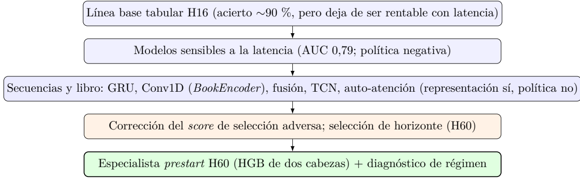
Figura 3.13: La escalera de modelos. Cada paso debe superar al anterior bajo el mismo protocolo; si no lo hace, se descarta.
