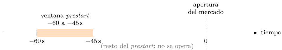
Figura 3.15: La ventana prestart del especialista: solo se opera entre -60 y -45 segundos respecto a la apertura del mercado, donde el análisis exploratorio detectó una densidad atípica de actividad del libro.
