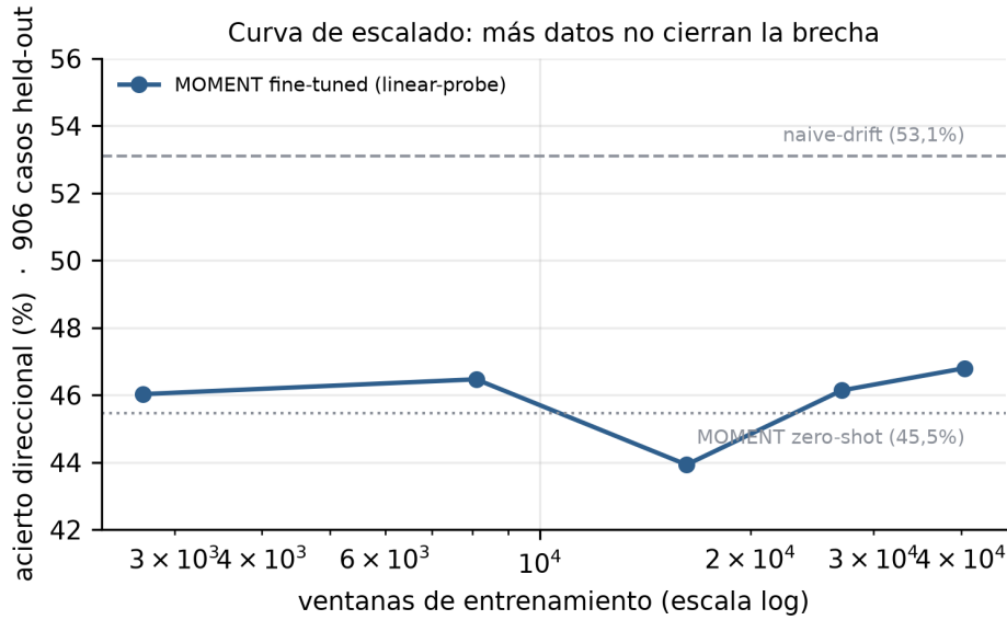
Figura 3.14: Curva de escalado del fine-tuning de MOMENT (linear-probing) frente al número de ventanas de entrenamiento, evaluada sobre los 906 casos congelados. Más datos no cierran la brecha con la deriva simple: el techo lo marca el régimen de datos, no el tamaño de la muestra.
