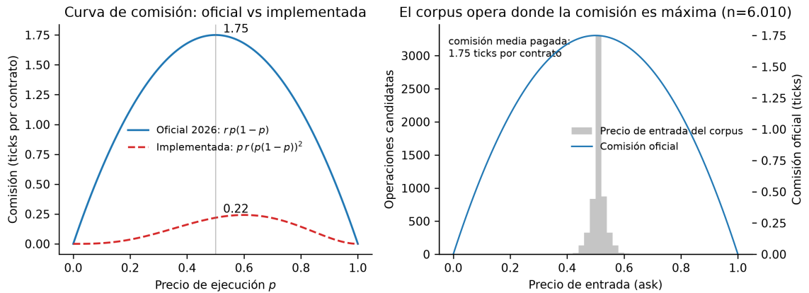
Figura 3.12: Fe de erratas del modelo de costes. Izquierda: comisión oficial de 2026 ( r p(1 - p) , r = 0,07 ) frente a la fórmula implementada originalmente, en ticks por contrato; en p = 0,5 la diferencia es de un factor ocho (1,75 frente a \sim 0,22 ). Derecha: distribución del precio de entrada del corpus operable de la ventana fuera de muestra ( n=6.010 operaciones candidatas) superpuesta a la curva oficial: las operaciones se concentran precisamente donde la comisión es máxima, con un coste de entrada medio de 1,75 ticks por contrato.
