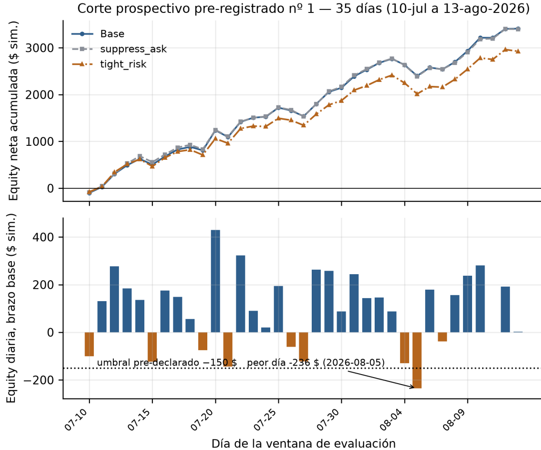
Figura 4.3: Corte prospectivo pre-registrado n° 1. Arriba, equity neta acumulada por brazo sobre los 35 días de la ventana. Abajo, equity diaria del brazo base con el umbral pre-declarado de -150\$ : el corte no falla por rentabilidad —la curva acumulada termina en +3.408\$ — sino por la profundidad de un único día, el 5 de agosto.
