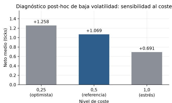
Figura 2: Sensibilidad al coste del subconjunto de baja volatilidad. Resultado exploratorio obtenido tras inspeccionar el mismo bloque.
