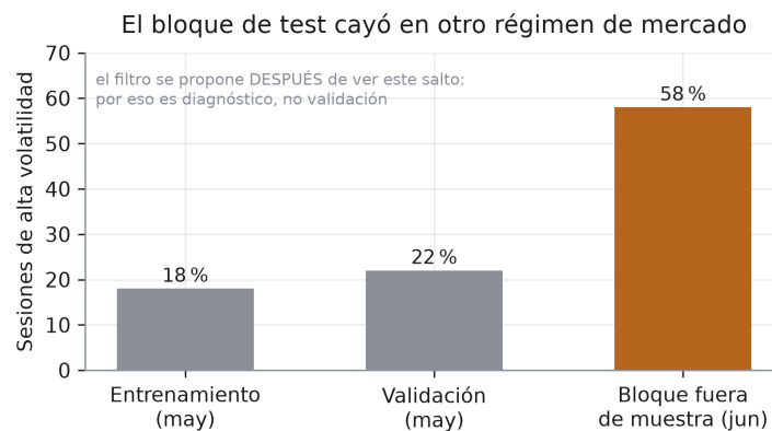
Figura 4.1: Fracción de sesiones de alta volatilidad por periodo. El salto del bloque nuevo motiva el análisis de régimen, pero no valida por sí mismo el filtro.
