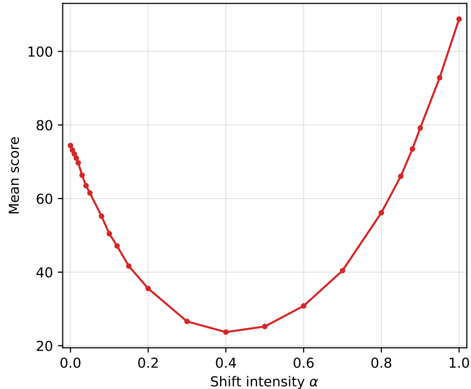
KL Text
