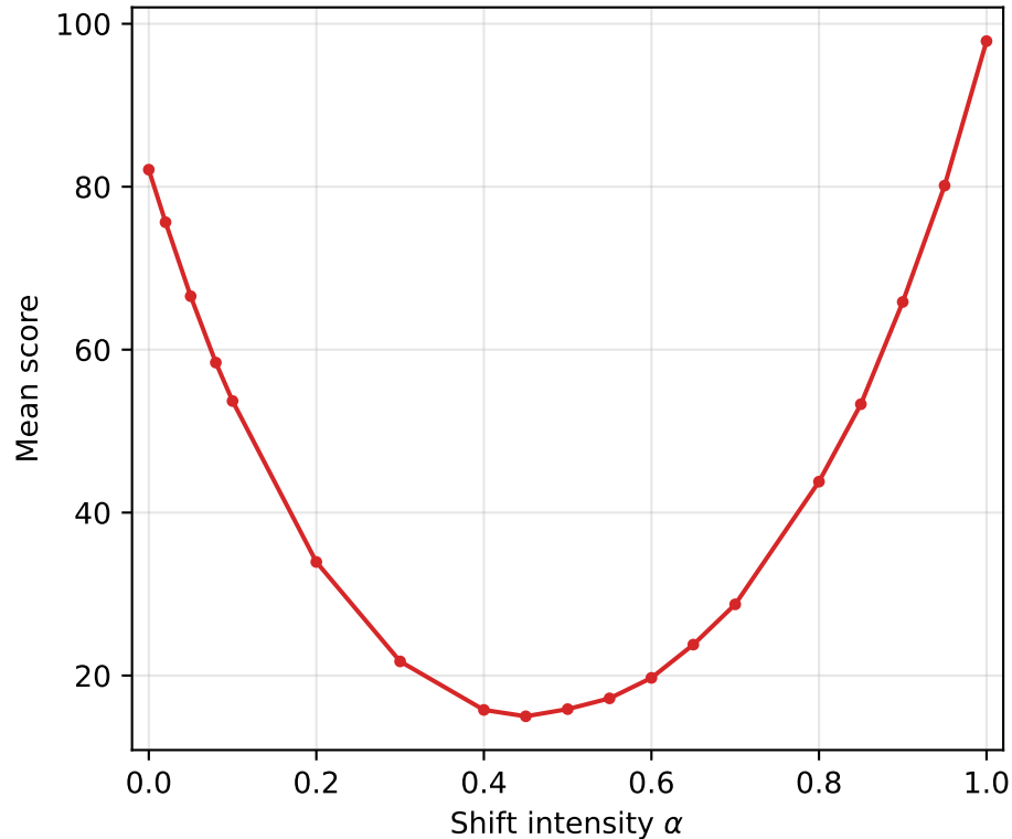
KL CIFAR-10
