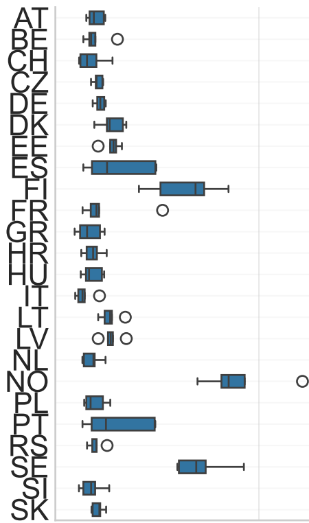
smape
