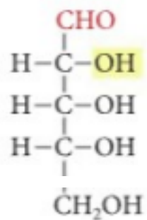
ribosio
