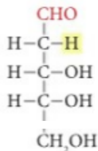
desossiribosio
