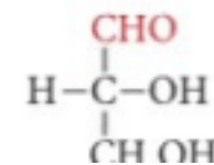
\text{CH}_2\text{OH} gliceraldeide
