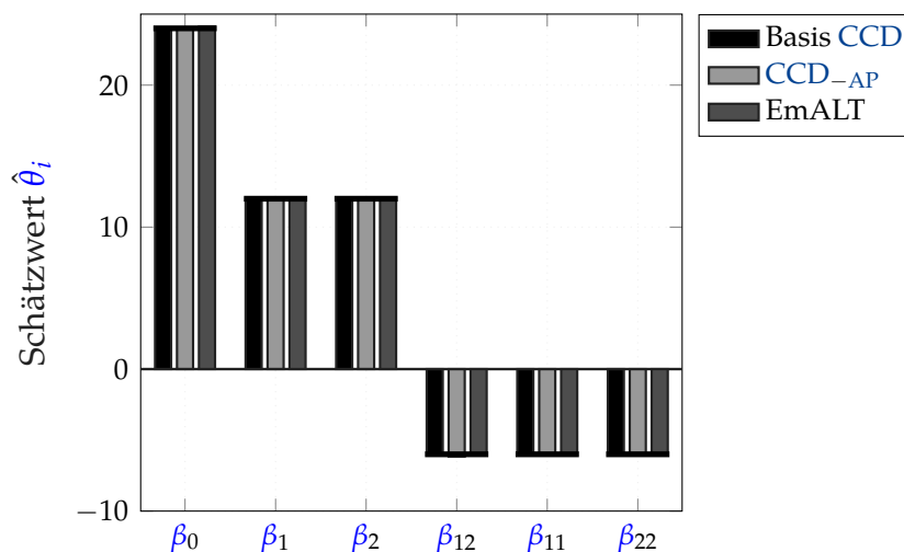
Abbildung 5.15: Absolute Schätzwerte der Modellkoeffizienten für die asymmetrischen Designvarianten am Arbeitspunkt \text{SNR} = 1,20 . Der Bias bleibt marginal; die Erwartungstreue des OLS-Schätzers ist gewahrt.
