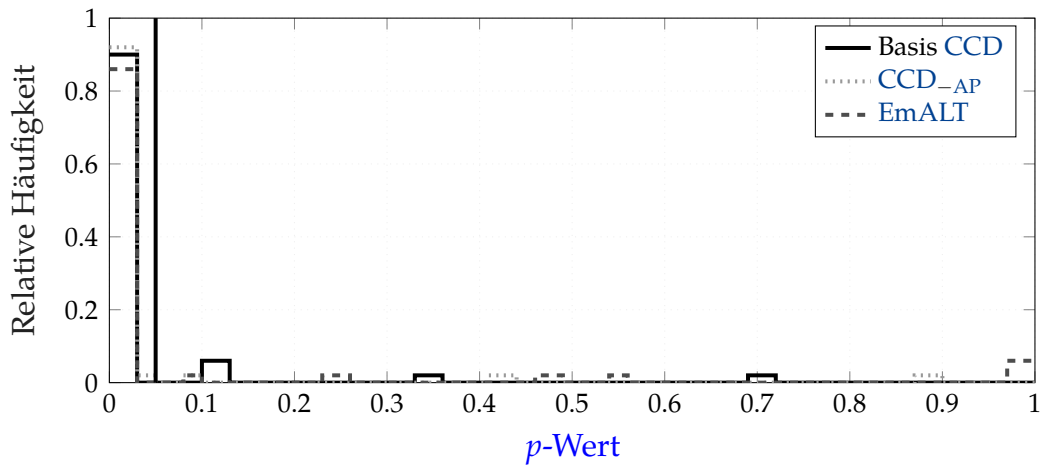
Abbildung 5.19: Aggregierte p -Wert Histogramme der MLE-Signifikanztests. Die stochastische Auswertung liefert artefaktfreie Verteilungen.
