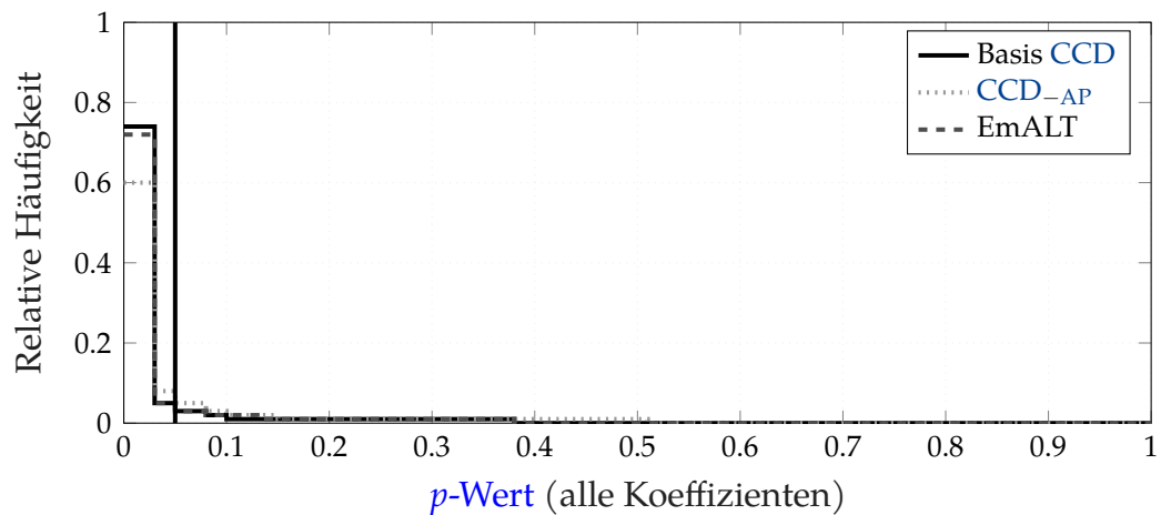
Abbildung 5.16: Aggregierte p -Wert Histogramme der verglichenen Designvarianten. Der konforme Verlauf belegt die Abwesenheit systematischer Verzerrungen in der Signifikanzprüfung.
