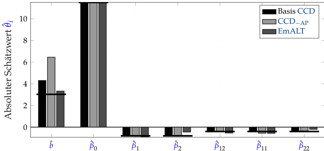
Abbildung 5.18: Absolute Schätzwerte der MLE-Koeffizienten im Weibull-Modell ( \text{SNR} = 1,20 ). Die Asymmetrie des EmALT provoziert keine unzulässigen systematischen Verzerrungen.
