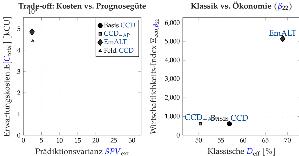
Abbildung 5.21: Ökonomisch-statistischer Trade-off: Gegenüberstellung von Erwartungskosten \mathbb{E}[C_{\text{total}}] , Prädiktionsvarianz SPV_{\text{ext}} und klassischer D-Effizienz.
