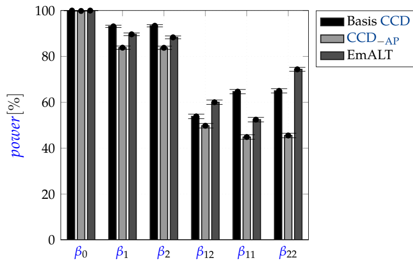
Abbildung 5.17: Vergleichende Analyse der absoluten statistischen Trennschärfe. Die asymmetrische Extrapolationsabsicherung (EmALT) stellt die Detektionsrate im Vergleich zur reinen Ausdünnung nahezu vollständig wieder her.
