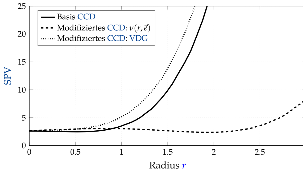
Abbildung 5.13: Der klassische VDG verschleiert den lokalen Design-Nutzen des um APs modifizierten CCD durch radiale Mittelung. Der EVG belegt hingegen die signifikante SPV -Reduktion zielgerichtet entlang des Extrapolationsvektors zum Prognosepunkt.
