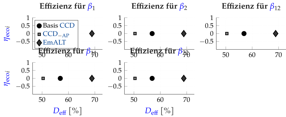
Abbildung C7: KPI ggü. D -Effizienz aller Koeffizienten.
