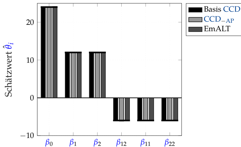
Abbildung 5.16: Absolute Schätzwerte der Modellkoeffizienten für die asymmetrischen Designvarianten am Arbeitspunkt \text{SNR} = 1,20 . Der Bias bleibt marginal; die Erwartungstreue des OLS-Schätzers ist gewahrt.
