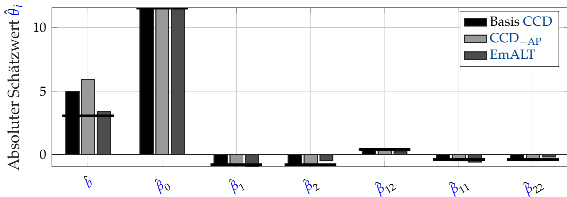
Abbildung 5.19: Absolute Schätzwerte der MLE -Koeffizienten im Weibull-Modell ( SNR = 1,20 ). Der Schätzwert der Basislebensdauer \hat{\beta}_0 bleibt exakt; die Terme höherer Ordnung spiegeln die durch die Multikollinearität induzierte Varianzumverteilung wider.
