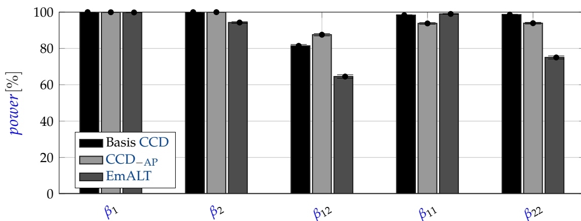
Abbildung 5.21: Vergleichende Analyse der MLE- power . Das EmALT-Design rettet die für die Modellierung essenziellen Terme vor dem vollständigen Zusammenbruch.
