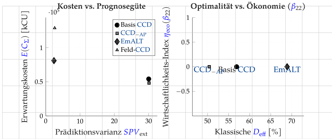
Abbildung 5.22: Links: Das Entkopplungs-Paradoxon als Pareto-Front zwischen Prädiktionsvarianz und Erwartungskosten. Das EmALT -Design funktioniert als ökonomisches Optimum. Rechts: Beweis des Versagens klassischer Optimalitätskriterien in der Zuverlässigkeitstechnik anhand des exemplarischen Verlaufs für den Krümmungsterm ( \beta_{22} ). Die scheinbar schlechteste D-Effizienz liefert den höchsten wirtschaftlichen Nutzen ( EPI, \eta_{eco\beta_{22}} ); die vollständige Evaluation aller Koeffizienten findet sich in Anhang C.2.
