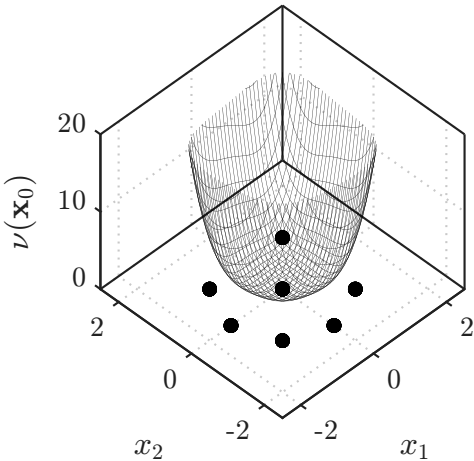
3D-SPV-Topologie
